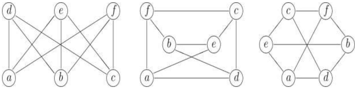
Рис. 11 – Изоморфные графы
