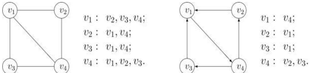
Рис. 12 – Примеры смежных вершин в графе
