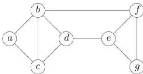
Рис. 14 – Пример маршрута, цепи и цикла в графе
