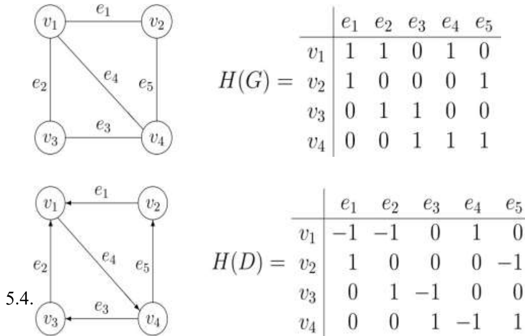
Рис. 13 – Примеры графов с соответствующими матрицами инцидентности
