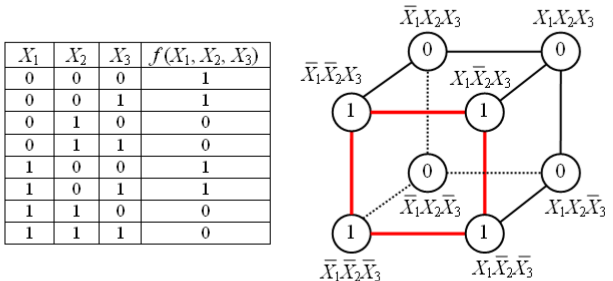
Рис. 4 - таблица истинности для булевой функции трех переменных и соответствующий ей куб
