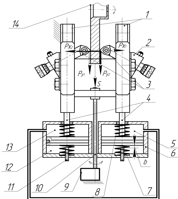
Рисунок – 3 Установка для обработки рабочих поверхностей тормозного диска: 1 – направляющая; 2 – резцедержатель; 3 – резец; 4 – шток; 5, 13 – полость гидроцилиндра с маслом; 6 – корпус; 7, 8 – пружина; 9 – привод подачи; 10 – винт подачи; 11 – регулировочный винт; 12 – полость; 14 – тормозной диск
