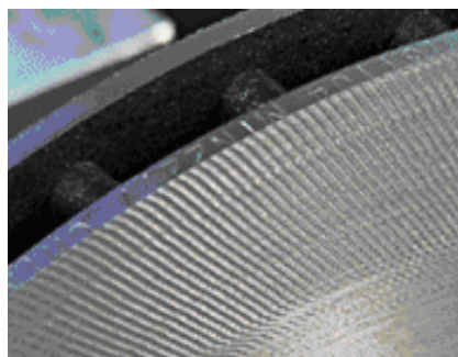
Рисунок 2 – Рабочая поверхность тормозного диска при появлении резонансных вибраций во время обработки
