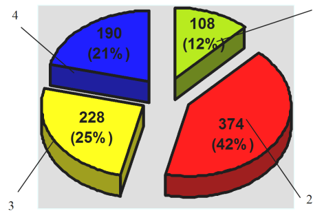
Рисунок 1 – Результаты тестирования тормозной системы 900 автомобилей различных марок и моделей:
