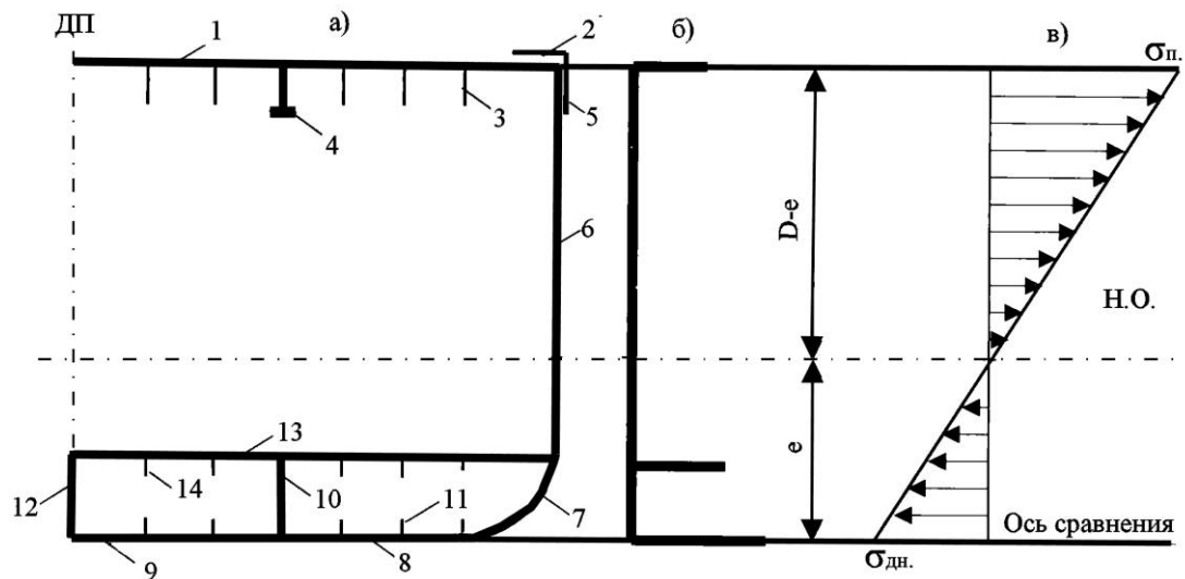
Рис. 2.1. Схема поперечного сечения корпуса судна:
