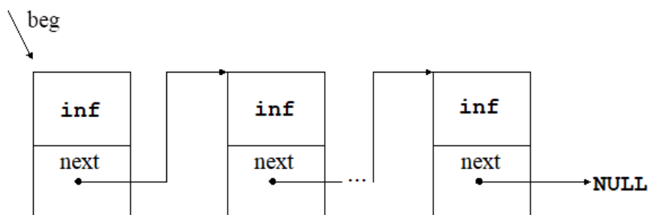
Рисунок 3.1 – Линейный список
