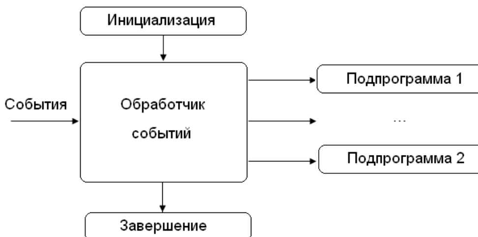
Рисунок 6.1 – Структура программы, управляемой событиями
