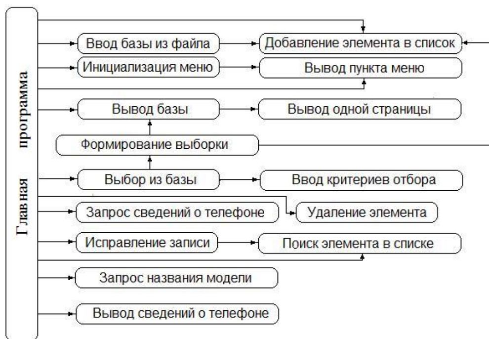
Рисунок 6.2 – Модульная структура программы
