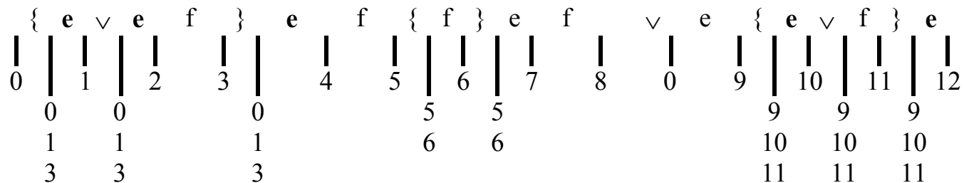
а) Первоначальная разметка регулярного выражения
