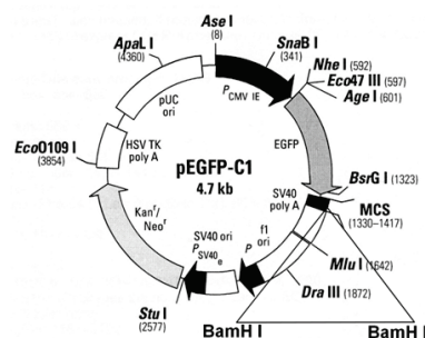
Рисунок 1. А. Структура «базового» вектора. Обозначено положение вводимого в состав плазмиды «модифицирующего» фрагмента ДНК (BamH I - BamH I). Б. Структуры «модифицирующих» вставок ДНК, клонированных в составе «базовой» плазмиды pEGFP-C1. Приведена трансляция 3'-концевой части гена GFP, жирным шрифтом выделены сайты BamHI, курсивом – поли-Г участки в структуре «модифицирующих» вставок ДНК
