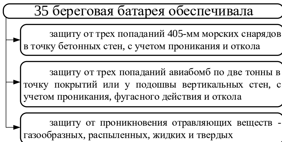
Рисунок 2 – Оперативно-технические характеристики 35 береговой батареи на момент приемки в 1929 году
