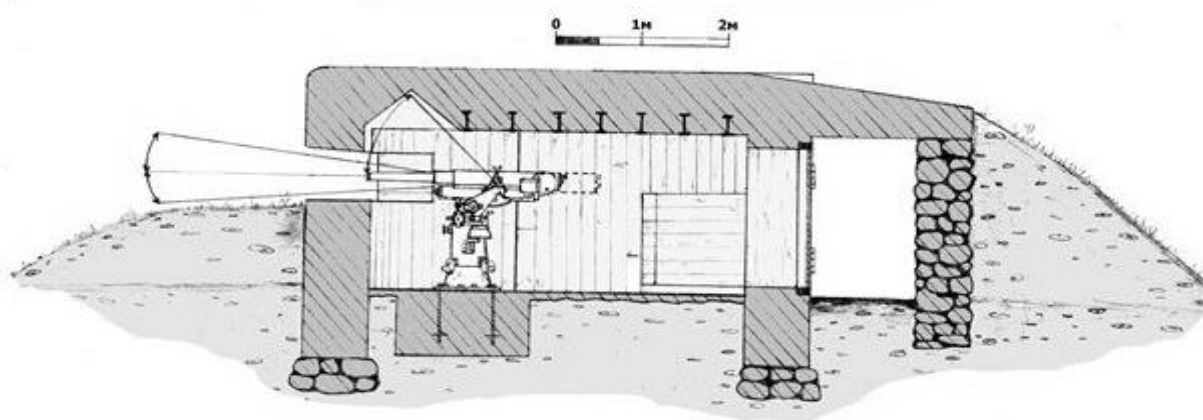
Рисунок 3 – Схема построения артиллерийского ДОТа №20 [5]
