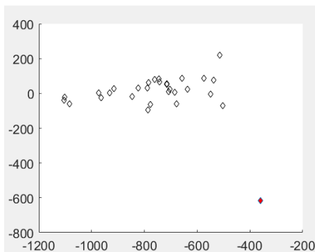
Рис. 15. Новая пара, красный ромбик — сильный аутлаер.
