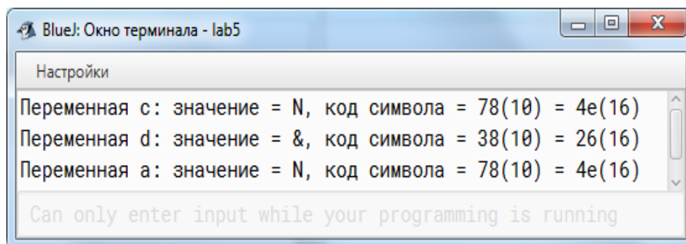
Рисунок 6.6 – Результат выполнения программы на тесте 4
