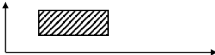
Рисунок 6.3. Область истинности выражения
