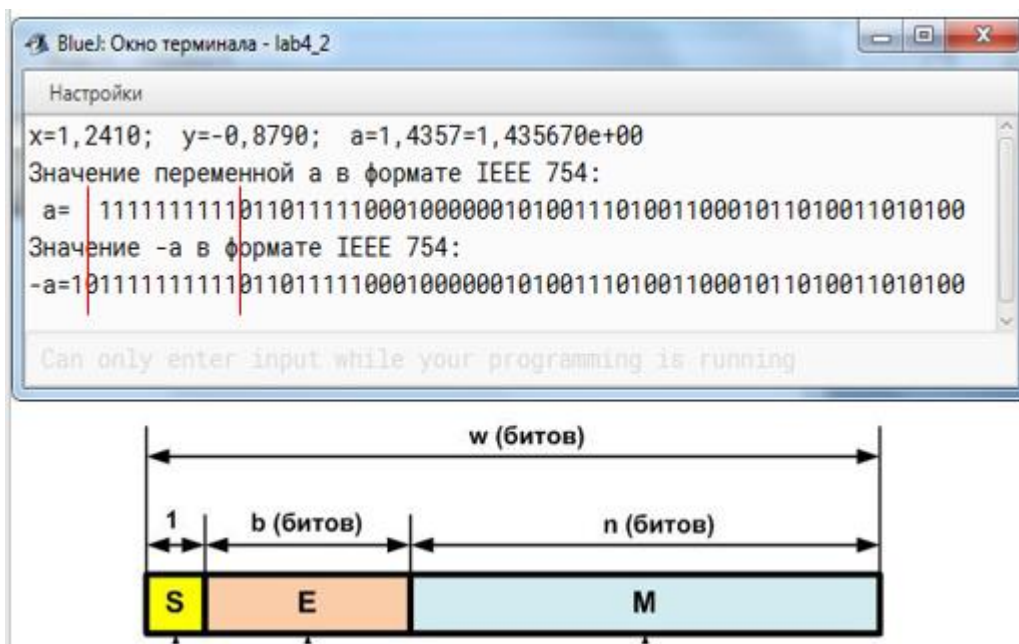
Рисунок 5.6 – Результаты вычислений и формат для их интерпретации
