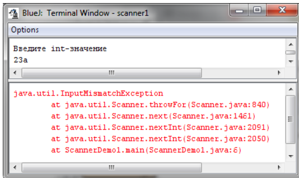
Рисунок 2.3 – Аварийное завершение программы
