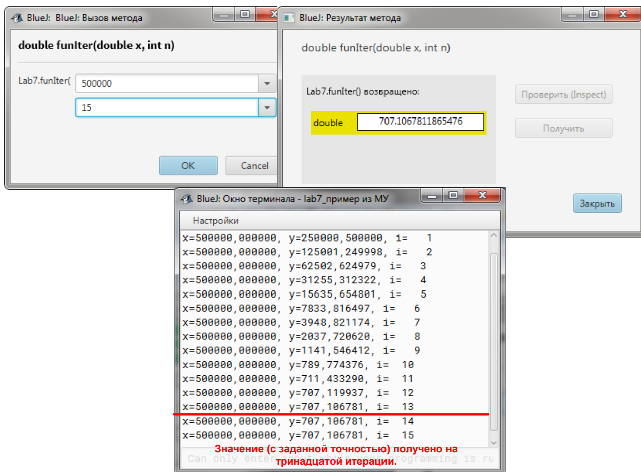
Рисунок 3.6 – Результаты вызова метода funIter(500000,15)
