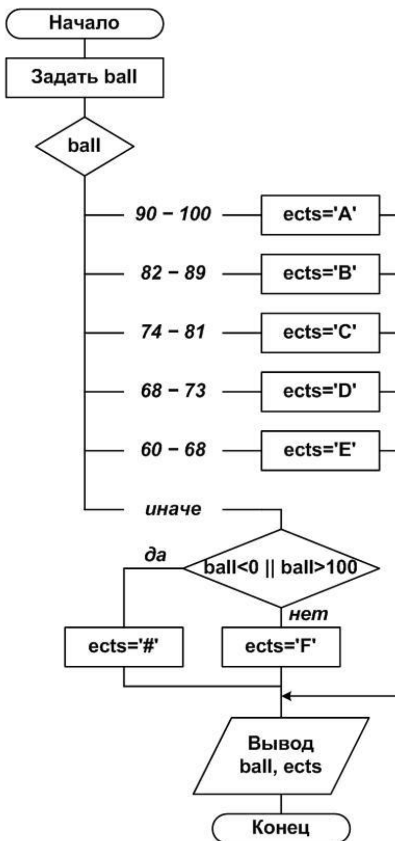
Рисунок 2.11 – Схема алгоритма перевода балльной оценки в оценку ECTS
