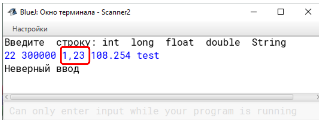
Рисунок 2.5 – Результат выполнения программы при неправильно введенных исходных данных
