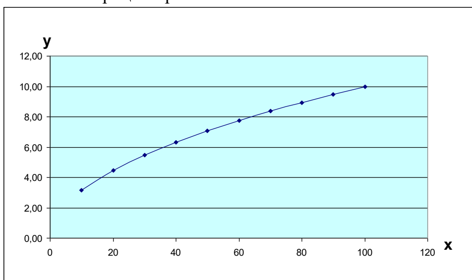
Рисунок 3.8 – График функции y = \sqrt{x} , построенный по результатам табулирования на интервале [10, 100] с шагом 10
