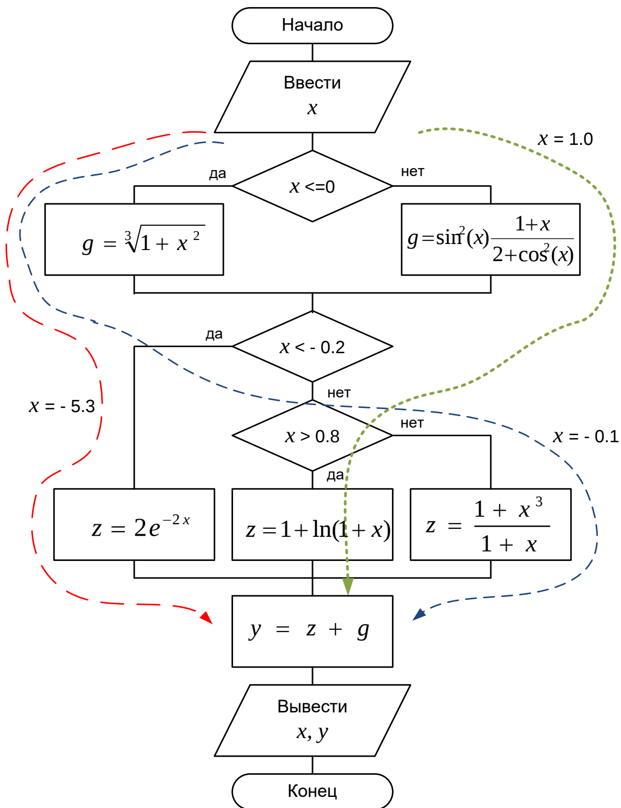
Рисунок 2.6 – Схема алгоритма и тестирования
