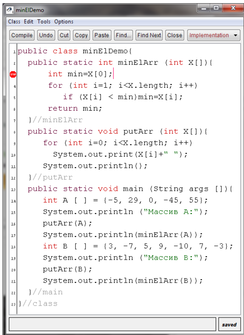
Рисунок 2.4 – Установка точки останова в программе
