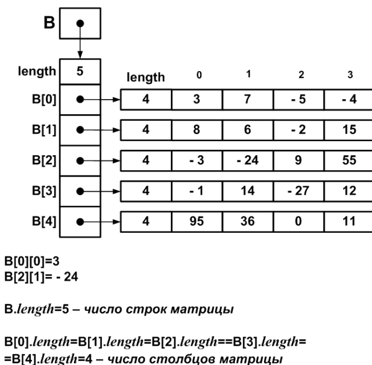
Рисунок 3.1 – Двумерный массив
