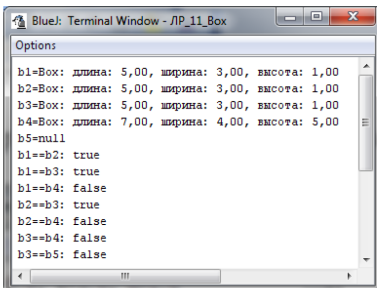
Рисунок 3.5 – Результаты выполнения программы
