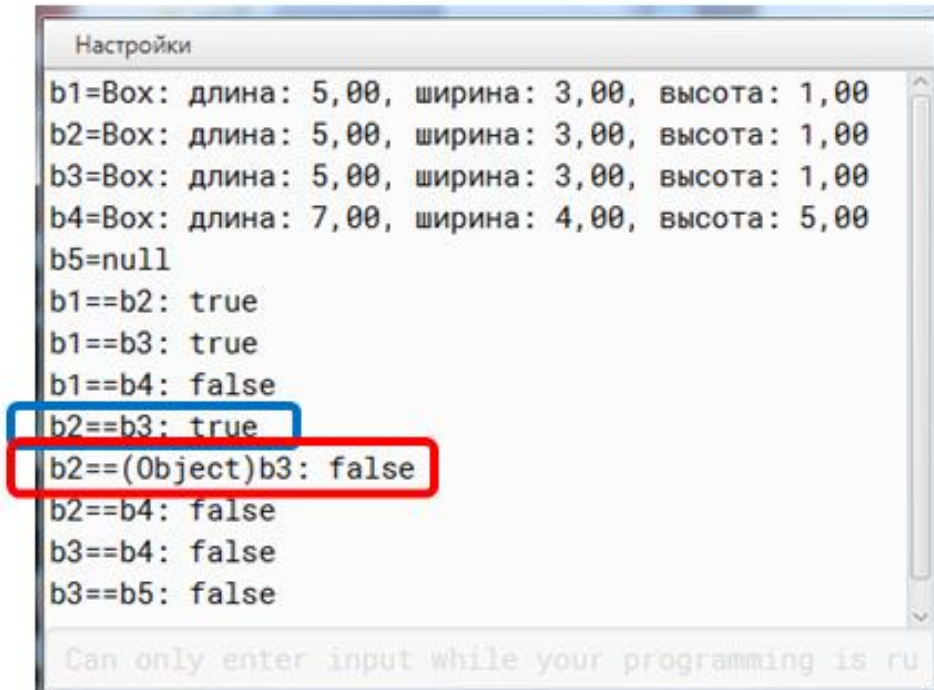
Рисунок 3.8 – Результаты вызовов перегруженных методов equals() при выполнении программы
