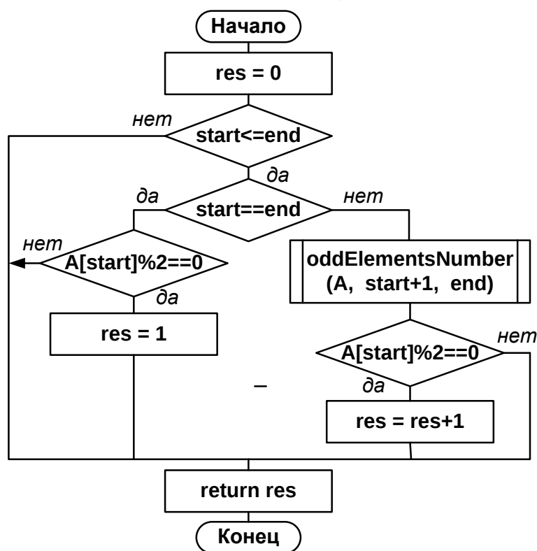
Рисунок 2.1 – Схемы алгоритмов: а) – рекурсивный метод; б) – итерационный метод
