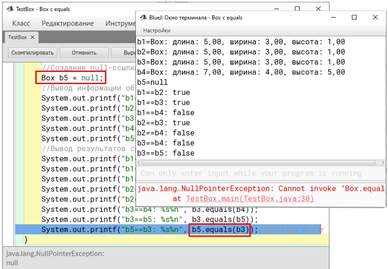
Рисунок 3.6 – Результат вызова экземплярного метода от имени null-ссылки
