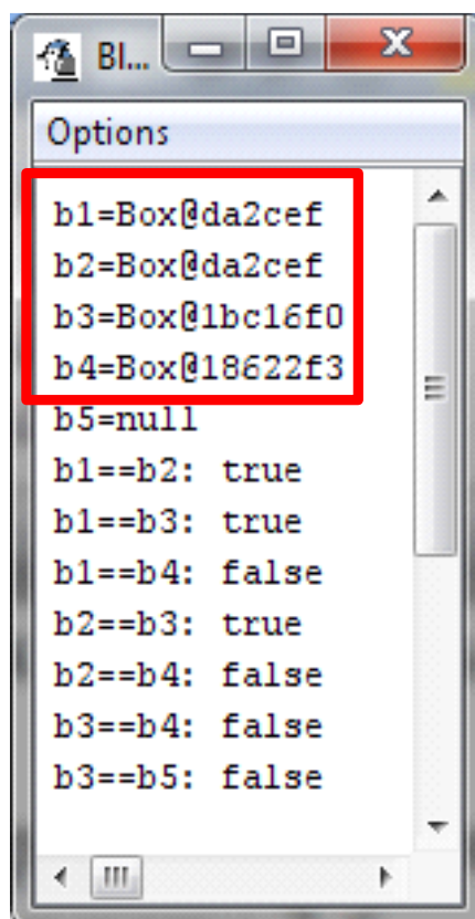
Рисунок 3.7 – Результаты выполнения программы при отсутствии в классе Box метода toString()
