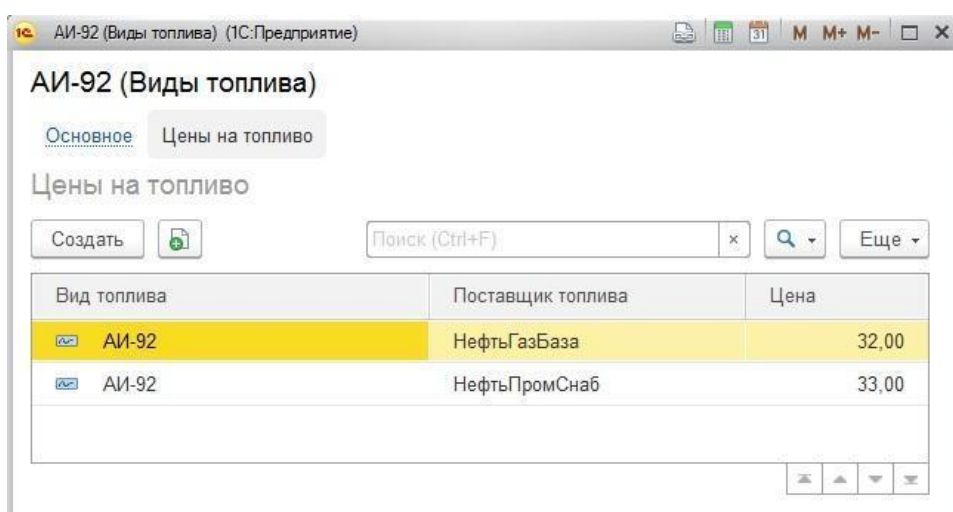
Рисунок 2.11 – Просмотр всех записей регистра
