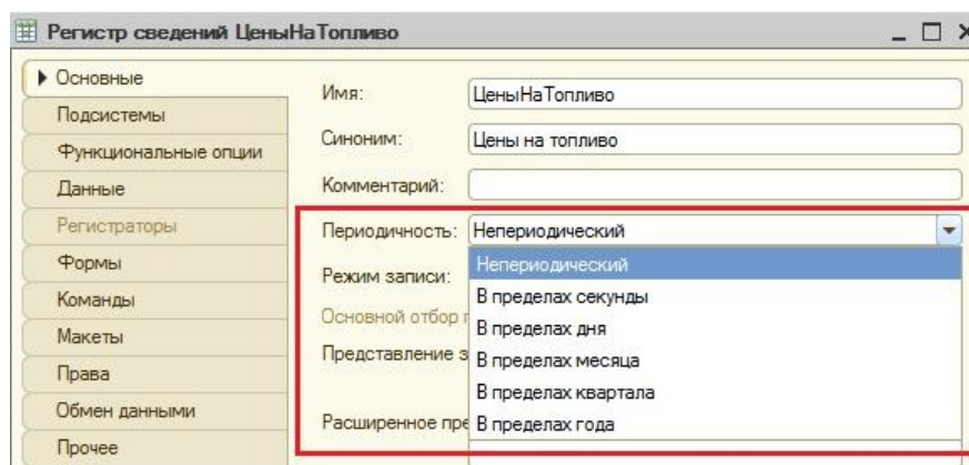
Рисунок 3.1 – Варианты определения периодичности регистра
