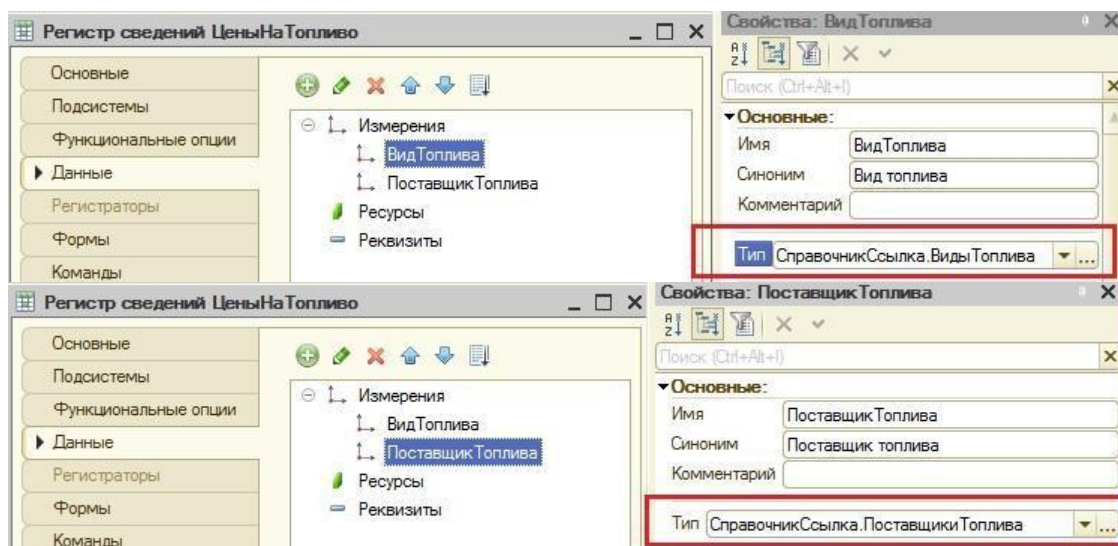
Рисунок 2.5 – Созданий измерений регистра сведений
