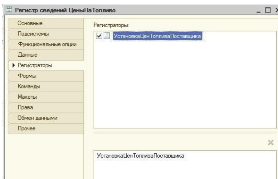
Рисунок 4.7 – Установка документа в качестве регистратора
