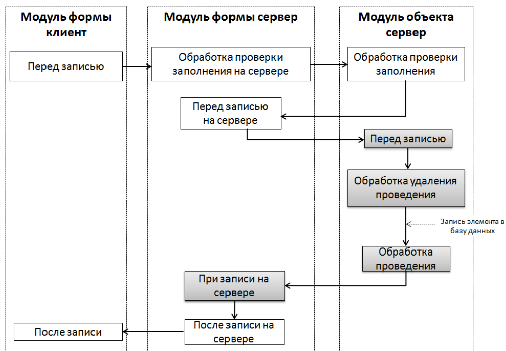
Рисунок 6.3 – Последовательность событий при отмене проведения документа
