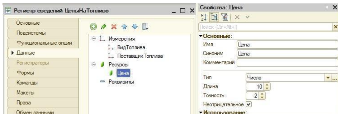
Рисунок 2.7 – Создание ресурса «Цена»
