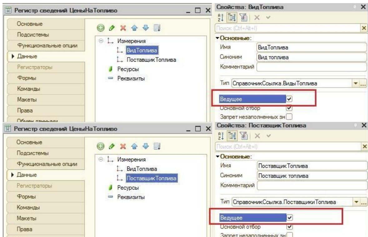
Рисунок 2.6 – Установка ведущих измерений регистра сведений
