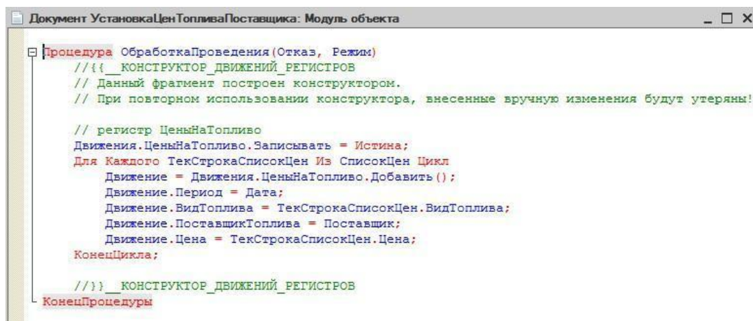
Рисунок 4.10 – Программный код, созданный конструктором движений
