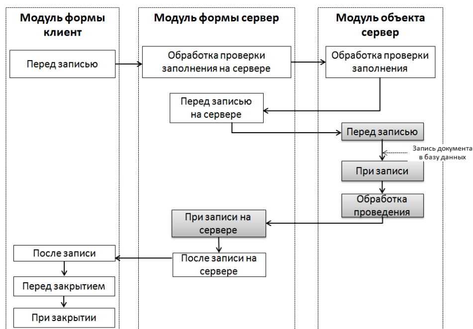
Рисунок 6.2 – Последовательность событий при проведении документа
