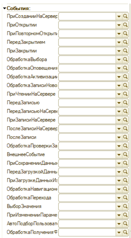
Рисунок 7.1 – Список обработчиков событий формы элемента справочника
