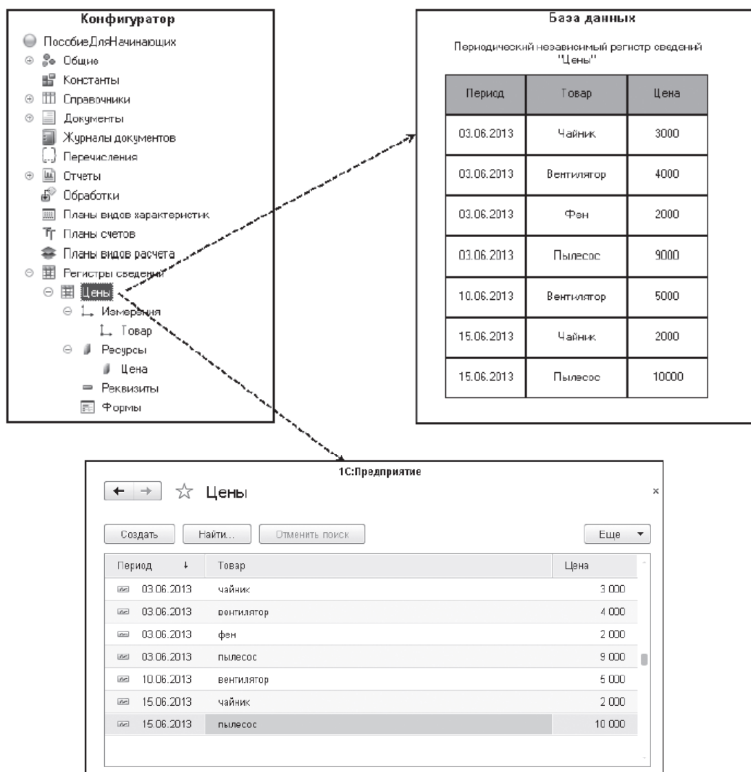
Рисунок 3.2 – Схема хранения данных в периодическом регистре сведений
