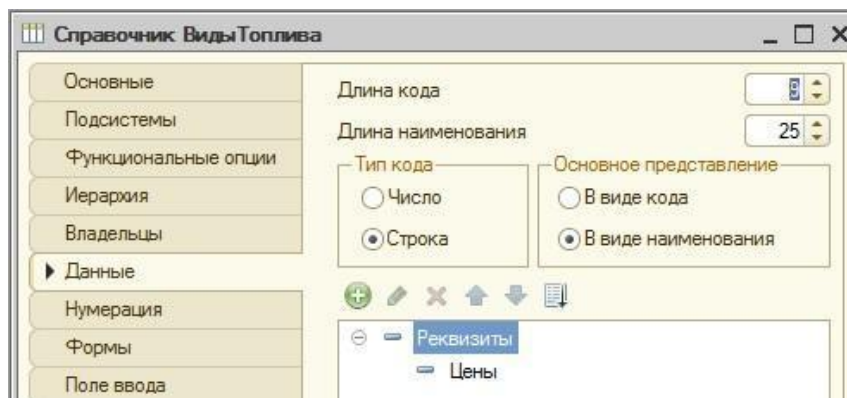
Рисунок 2.1 – Создание реквизита справочника
