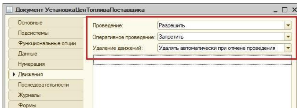
Рисунок 4.5 – Установка параметров движений документа
