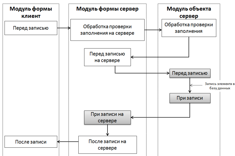
Рисунок 6.1 – Последовательность событий при записи документа
