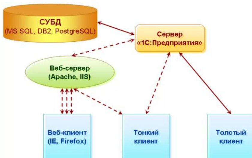
Рисунок 8.1 – Схема клиент-серверного взаимодействия
