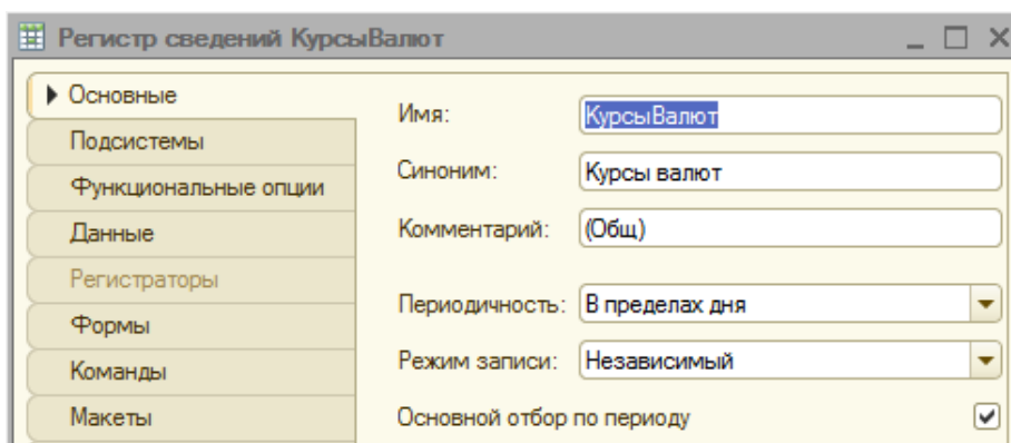
Рисунок 3.3 – Хранение курса валют с помощью регистра сведений
