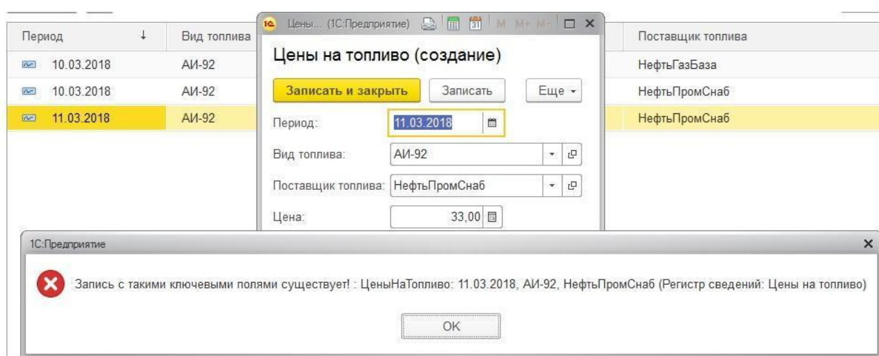
Рисунок 3.8 – Нарушение уникальности периода записей
