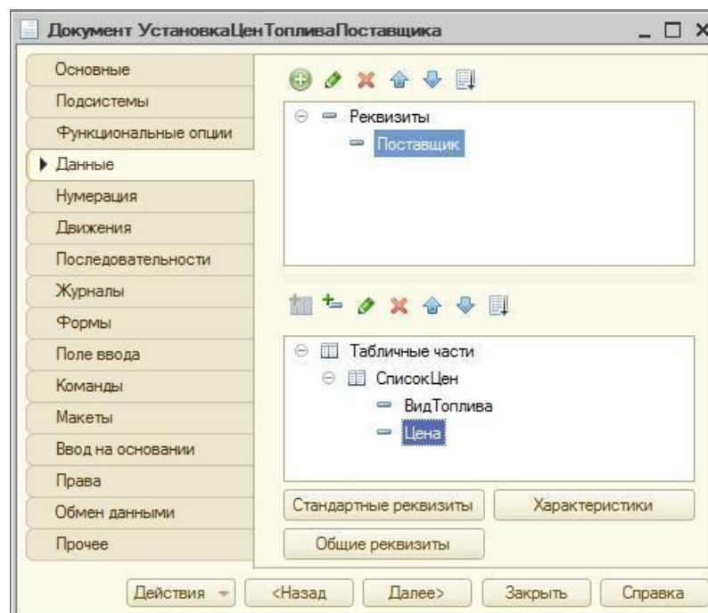
Рисунок 4.4 – Документ «Установка цен топлива»
