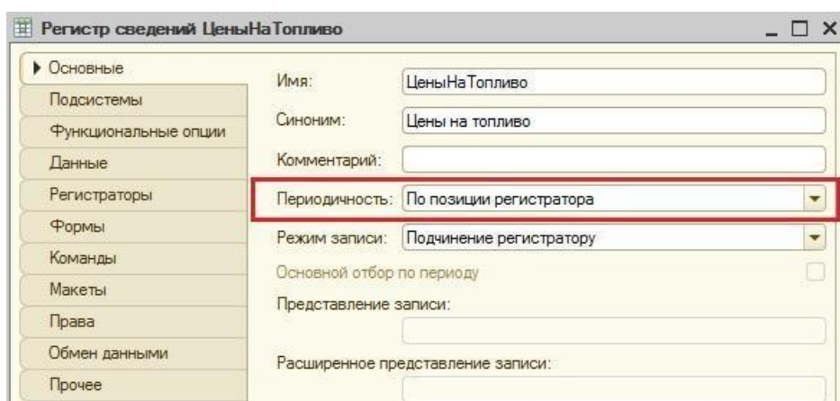
Рисунок 4.14 – Периодичность по позиции регистратора
