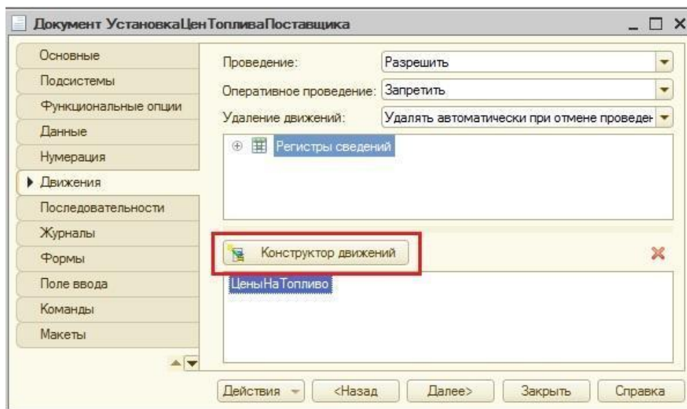
Рисунок 4.8 – Запуск конструктора движений
