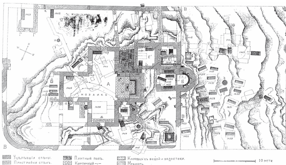
Рис. 3. План Херсонесского Загородного храма (Из отчета К.К. Косцюшко-Валюжинича в ИАК. Вып. 9).
