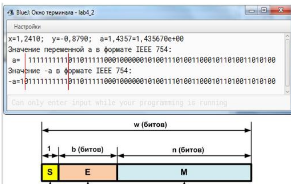
Рис. 5.6. Результаты вычислений и формат для их интерпретации
