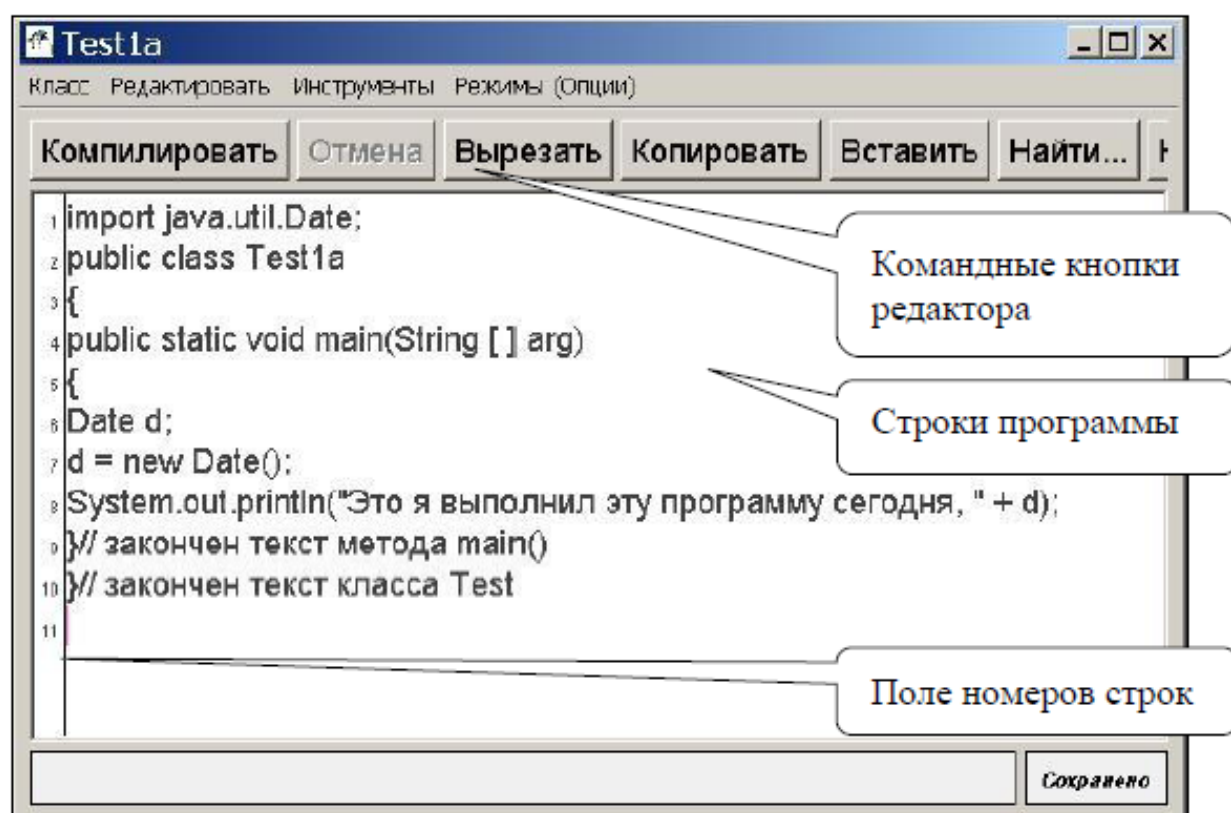
Рис. 2.3. Окно текстового редактора
