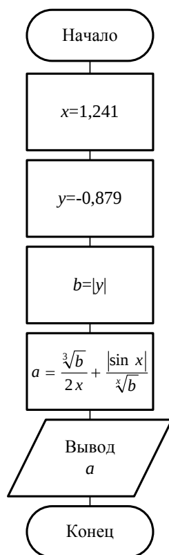
Рис. 5.5. Схема алгоритма вычислений
