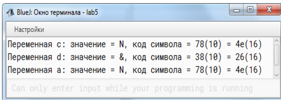
Рис. 6.7. Результат выполнения программы на тесте 4
