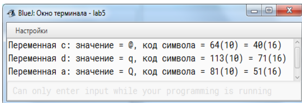
Рис. 6.5. Результат выполнения программы на тесте 2
