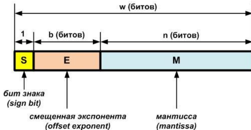
Рис. 5.1. Формат IEEE-754
