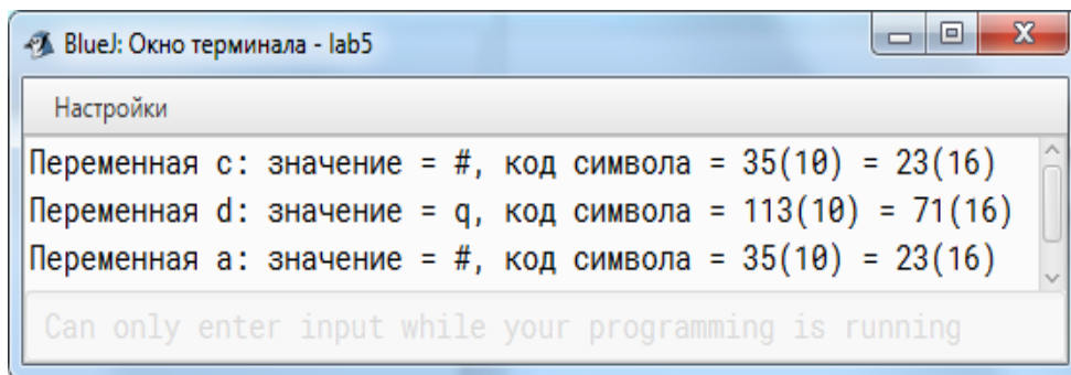
Рис. 6.6. Результат выполнения программы на тесте 3
