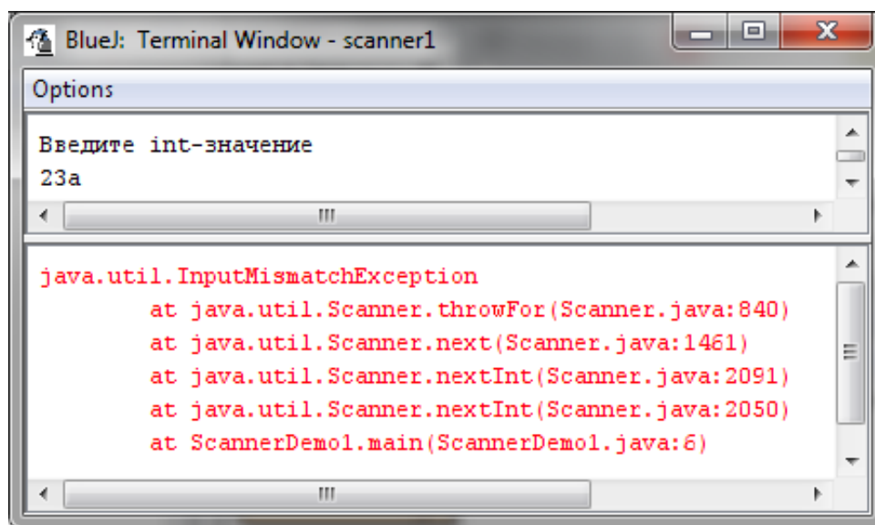
Рис. 2.3. Аварийное завершение программы
