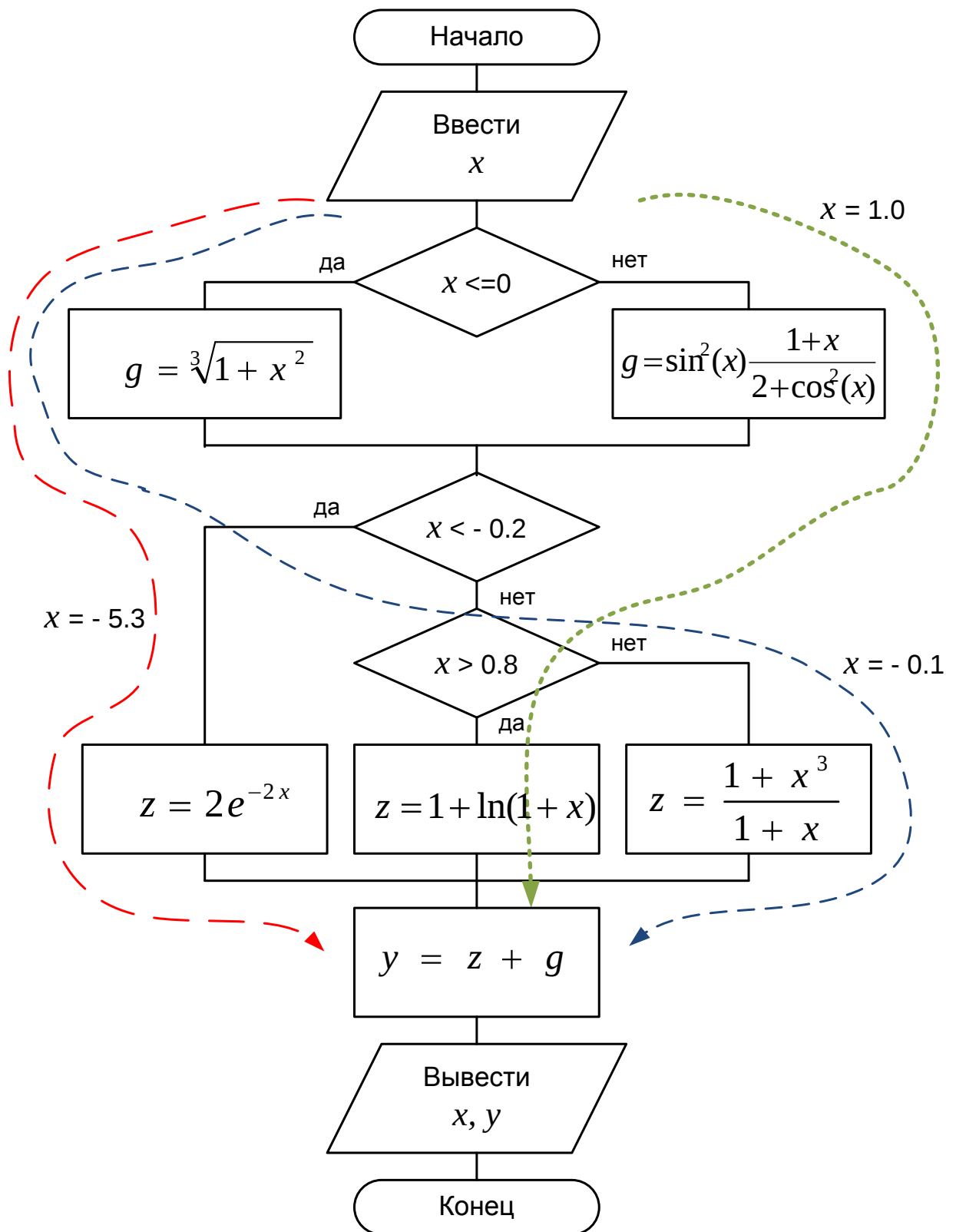
Рис. 2.6. Схема алгоритма и тестирования
