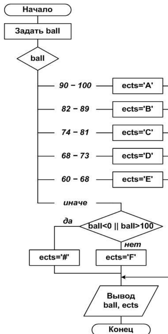
Рис. 2.11. Схема алгоритма перевода балльной оценки в оценку ECTS
