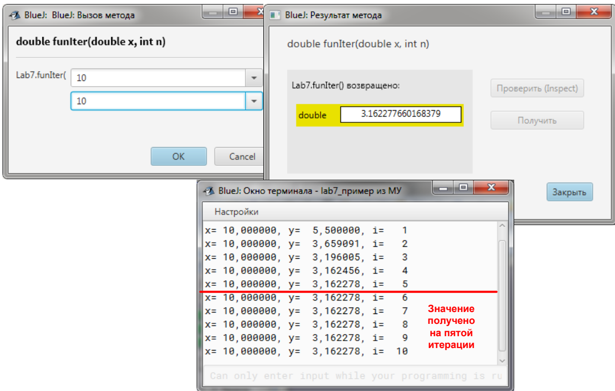
Рис. 3.5. Результаты вызова метода funIter (10,10)
