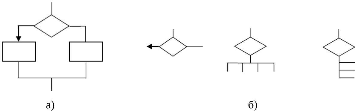
Рис. 2.1. Структура «ветвление» (а); изображение элементов для организации ветвления с двумя или несколькими альтернативами (б)
