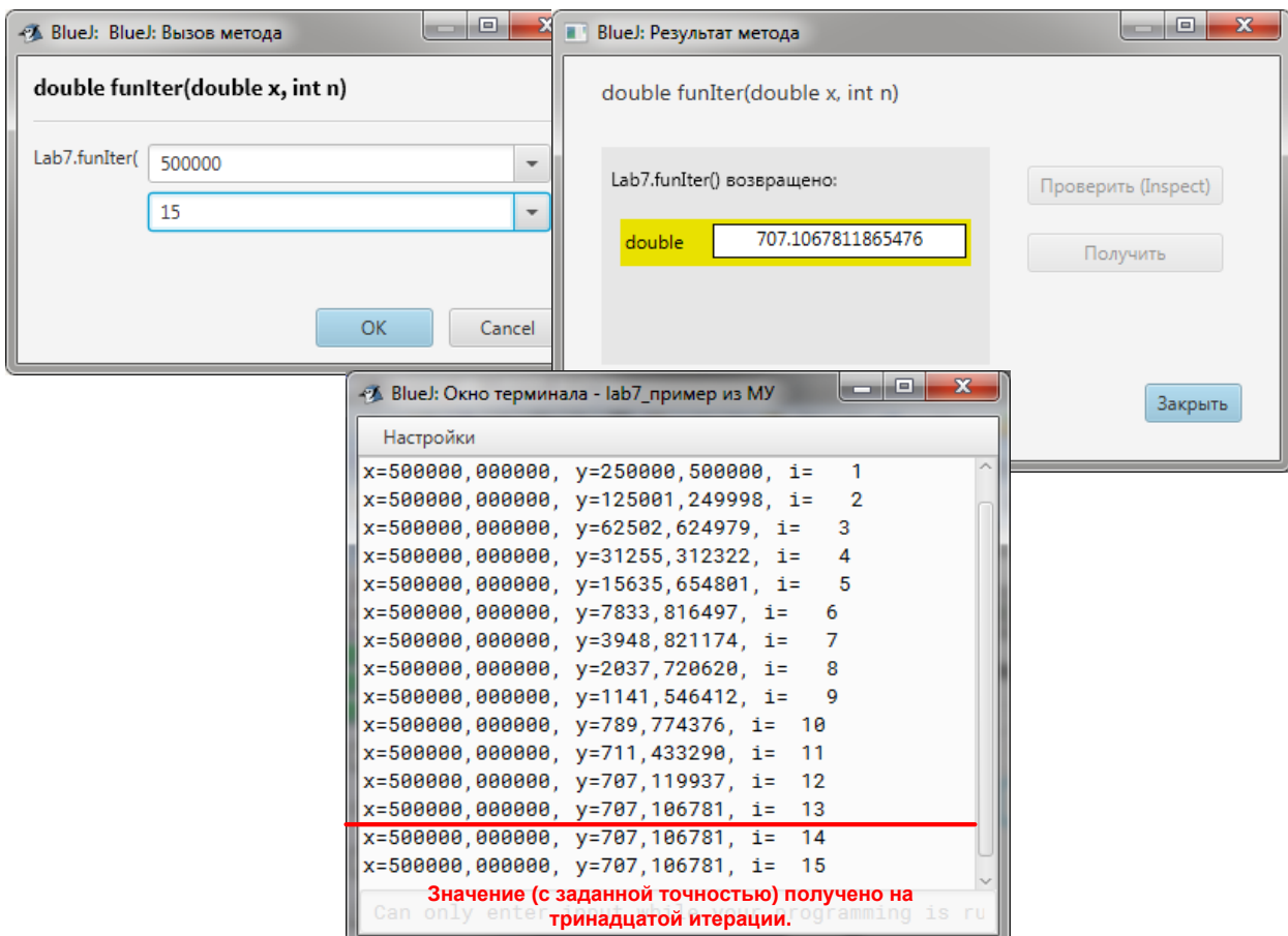
Рис. 3.6. Результаты вызова метода funIter (500000,15)
