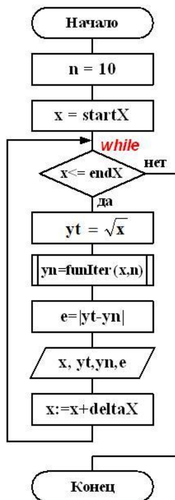
Рис. 3.4. Алгоритм табулирования функции
