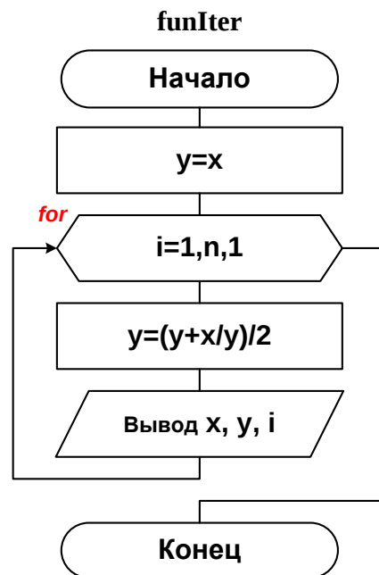
Рис. 3.3. Алгоритм вычисления корня по рекуррентной формуле
