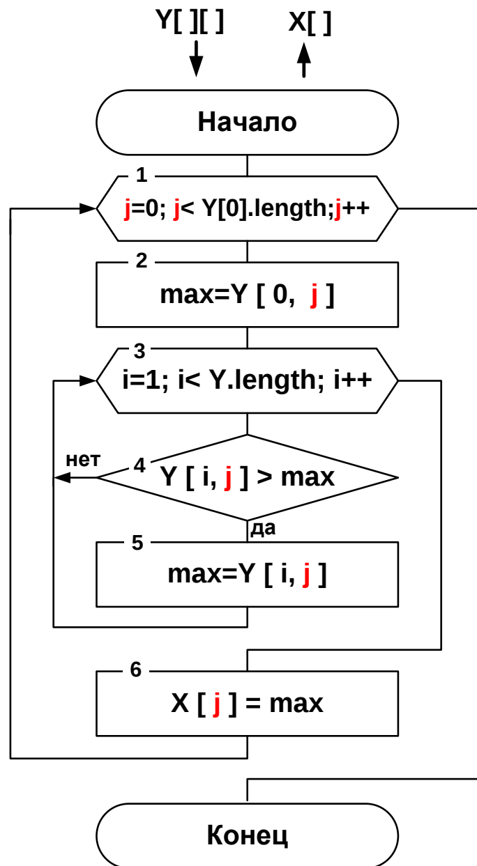
Рис. 3.2. Схема метода (функции) обработки массива
