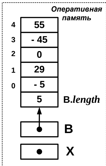
Рис. 2.2. Массив целых чисел B и пустая ссылка на массив целых чисел X
