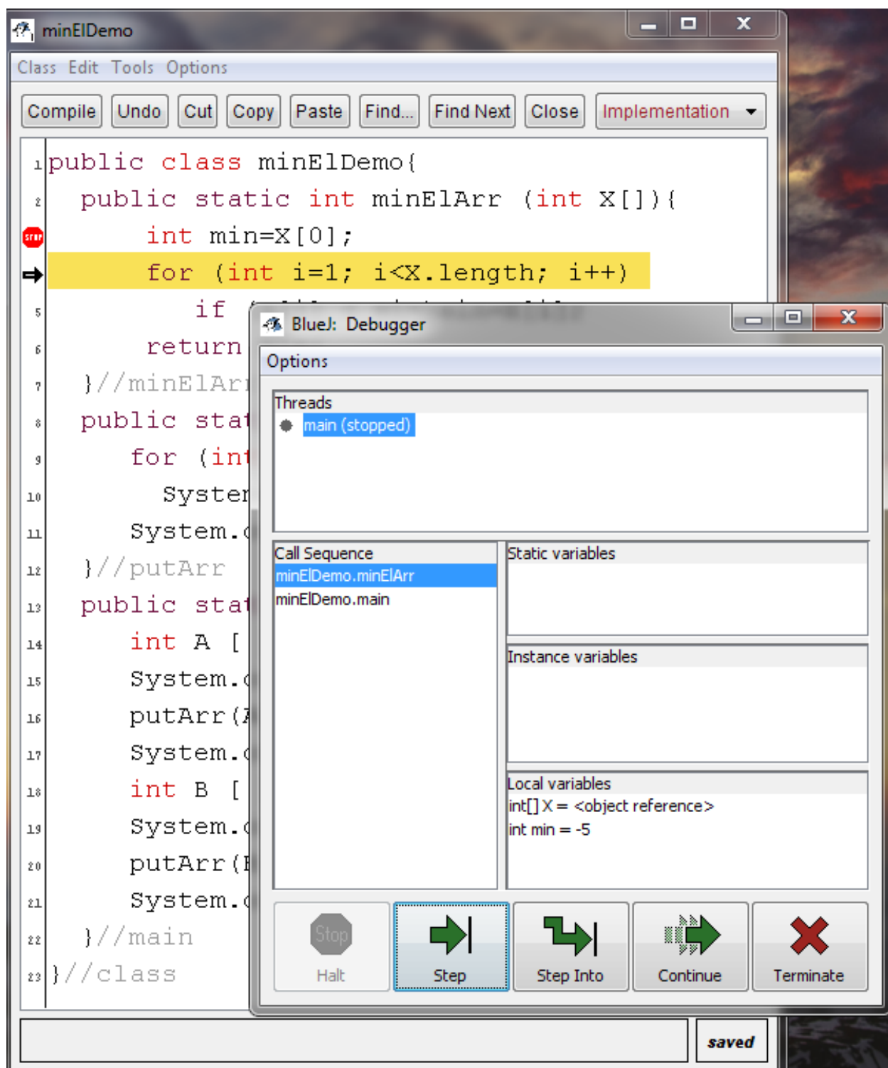
Рис. 2.7. Пошаговое выполнение (с точки останова) – шаг 1
