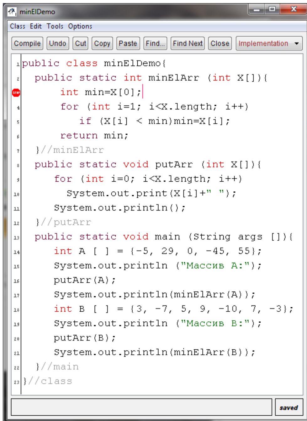
Рис. 2.4. Установка точки останова в программе
