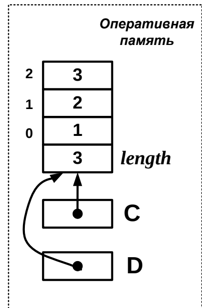
Рис. 2.3. Ссылки на один и тот же массив – синонимы C и D
