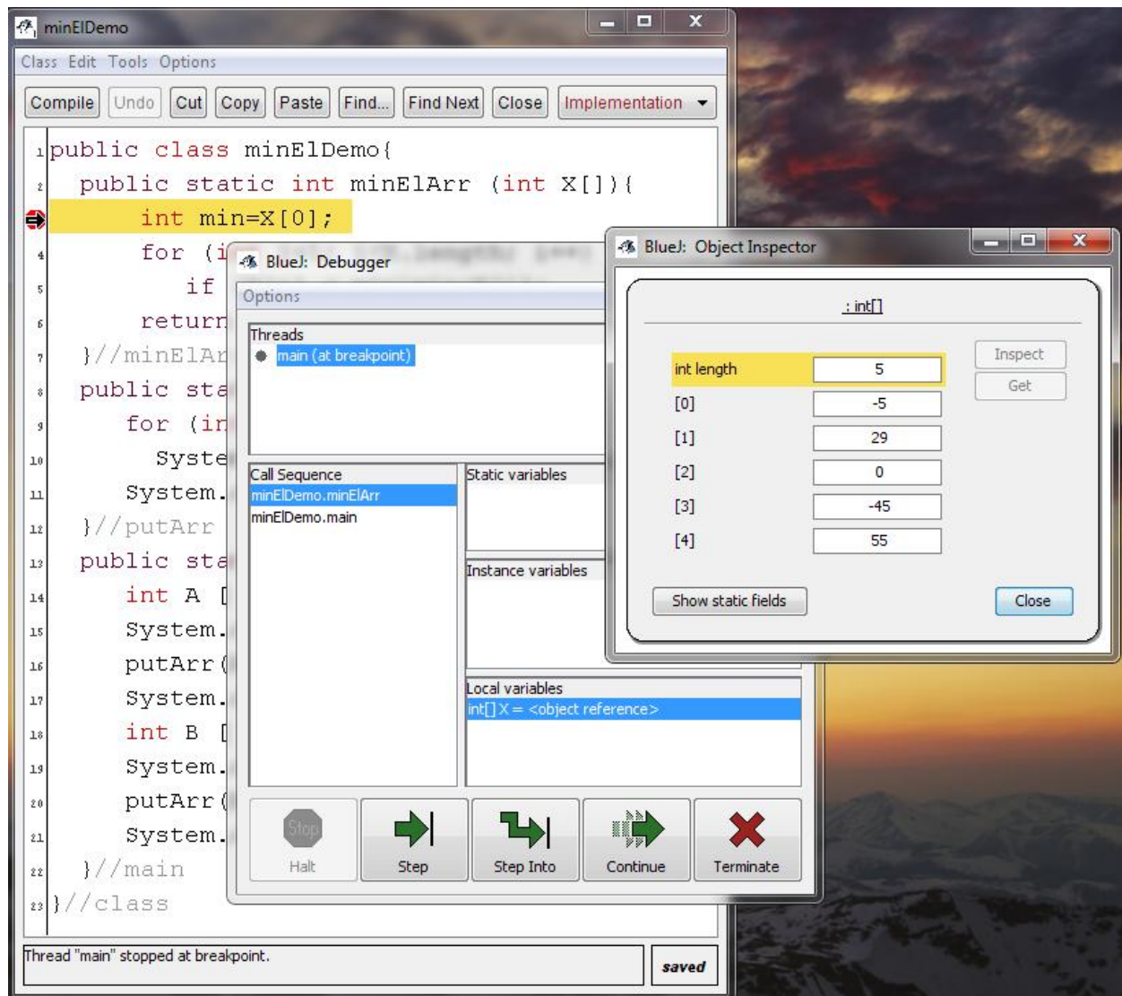
Рис. 2.6. Просмотр элементов массива
