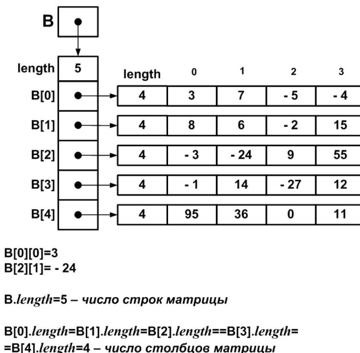
Рис. 3.1. Двумерный массив
