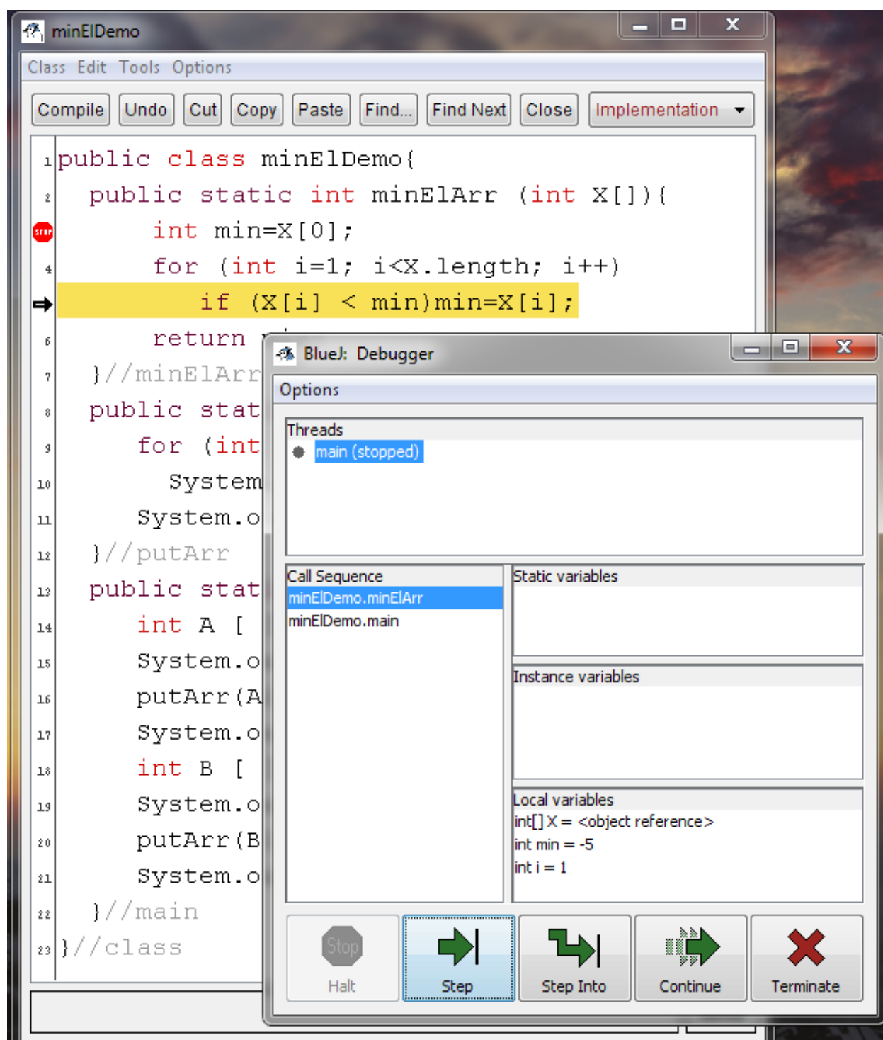
Рис. 2.8. Пошаговое выполнение – шаг 2
