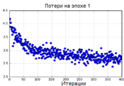
Рисунок 6 – Снижение потерь на одной эпохе для модели CNN
