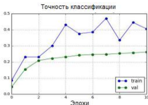
Рисунок 4 – Точность классификации 2-слойной полносвязной нейронной сетью с использованием признаков изображения
