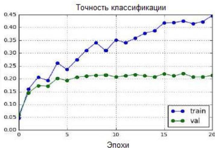
Рисунок 3 – Точность классификации для полносвязной 6-слойной нейронной сети
