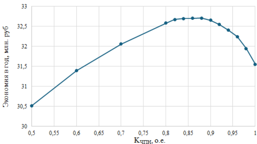
Рис. 4. Зависимость годовой экономии от коэффициента K_{чпн}
