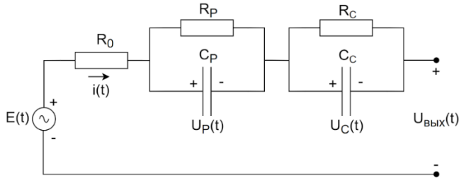
Рис 3. Схема замещения аккумулятора по DP-модели
