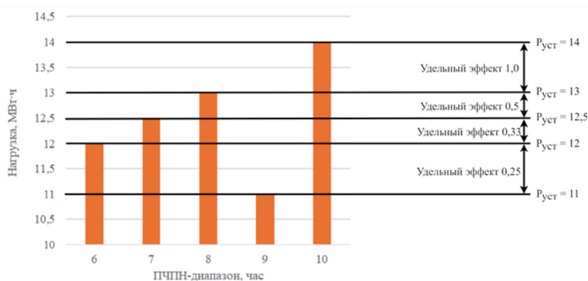
Рис. 5. Зависимость удельного эффекта алгоритма ПЧПН от уставки
