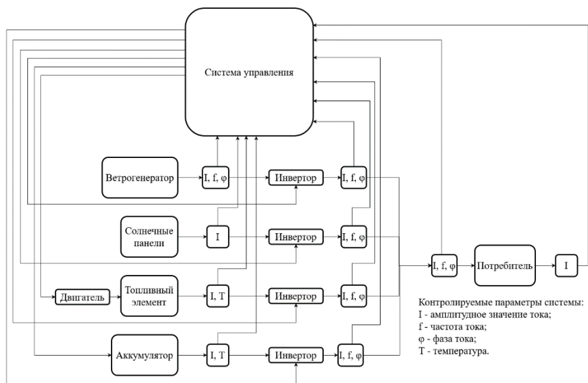
Рис.1. Структурная схема
