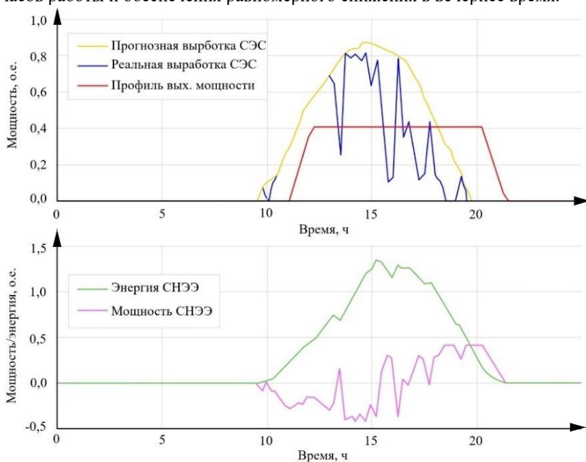
Рис. 1. График выработки электроэнергии СЭС на острове Ла-Реюньон с СНЭЭ энергоемкостью 9 МВт·ч
