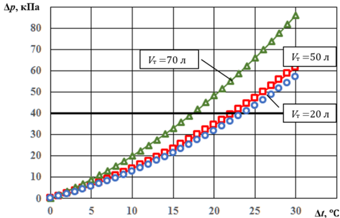
Рис. 5. Избыточное давление в баке ( p_{\text{р}} = 65 кПа)
