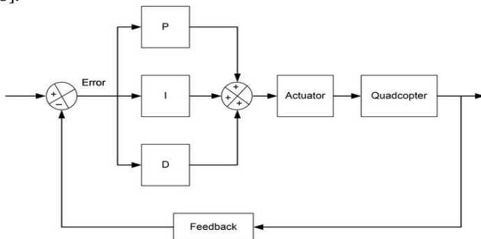
Рис. 2. Схема алгоритма работы системы управления
