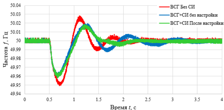
Рис. 5. Осциллограммы изменения частоты после изменения нагрузки в слабой сети с учетом настройки блока СИ
