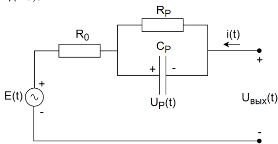
Рис 2. Схема замещения аккумулятора по модели Тевенина
