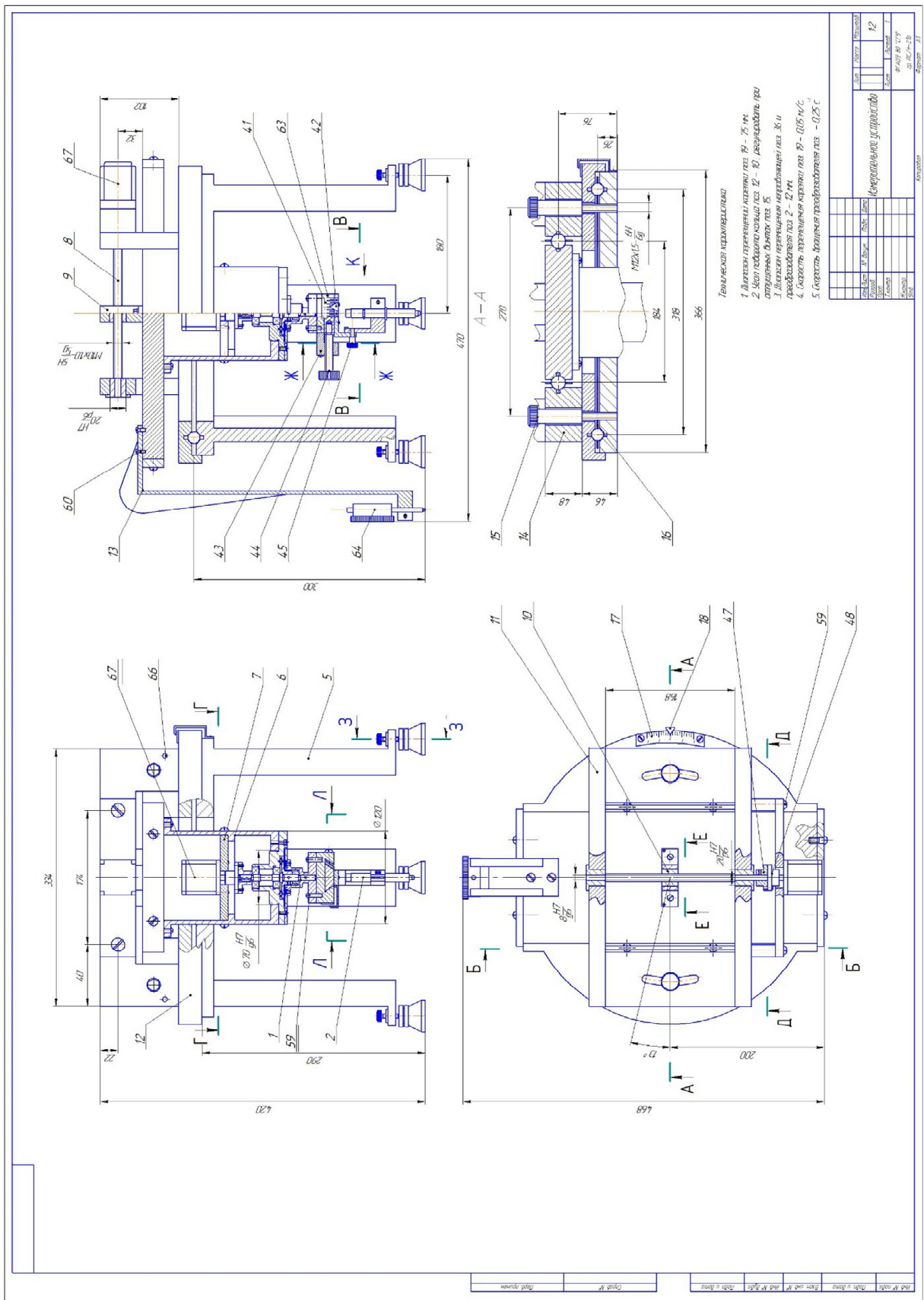
Рисунок А.5 – Измерительное устройство (сборочный чертёж)
