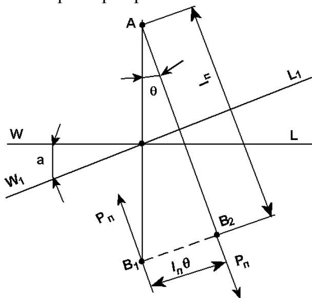
Рисунок 5.1 – Схема наклонения судна при подвешенном грузе
