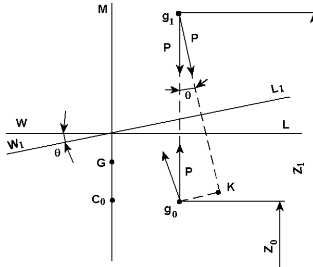
Рисунок 4.1 – Схема наклонения судна при переносе груза
