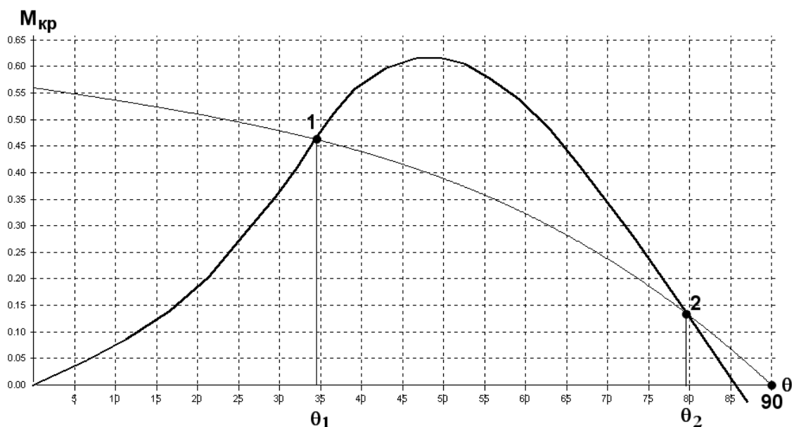
Рисунок 3.1 – Диаграмма статической остойчивости (пример)
