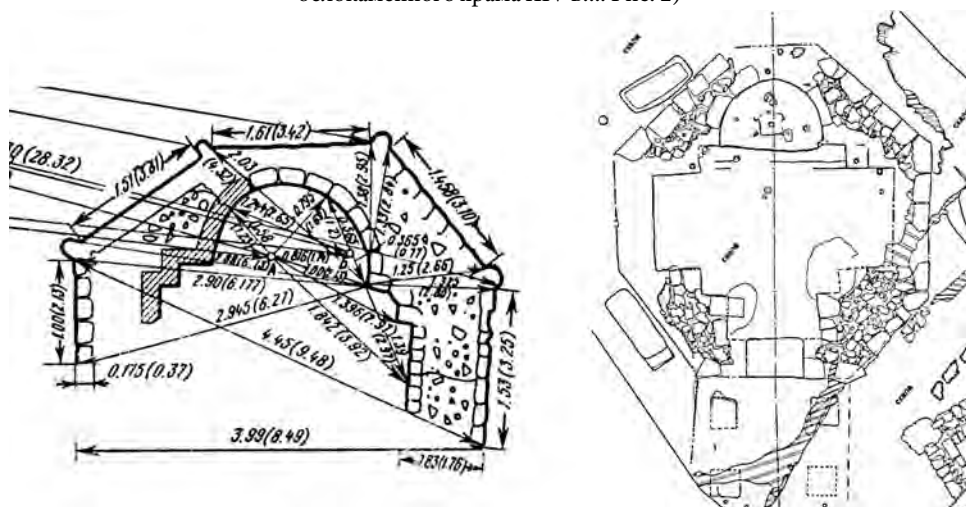
Рис. 4. Планы октагонов в Московском Кремле (Кавельмахер В.В., Рузаева Е.И.) и на Мангупе (Науменко В.Е., Герцен А.Г.)
