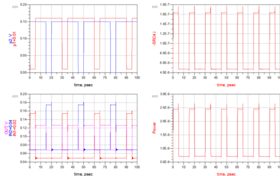
Рис. 14. Результаты моделирования схемы, представленной на рис. 13.
