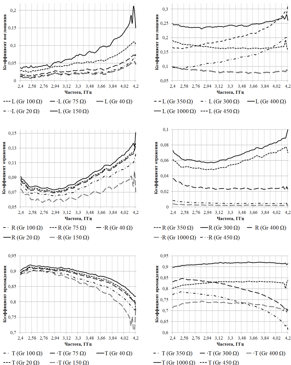
Рис. 4. Полученные значения коэффициентов: прохождения, отражения, поглощения образцов графена.
