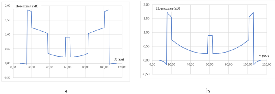
Рис. 16. Потенциальные рельефы для электронов в ячейке памяти на основе пересекающихся нанопроводов при нулевых смещениях: а — вдоль «тонкого» нанопровода; б — вдоль «толстого» нанопровода.
