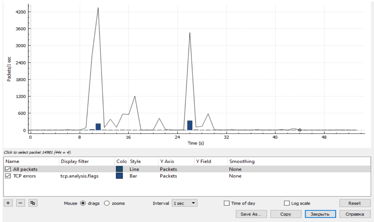
Рисунок 5.7 – График зависимости пропускной способности сети во время захвата трафика
