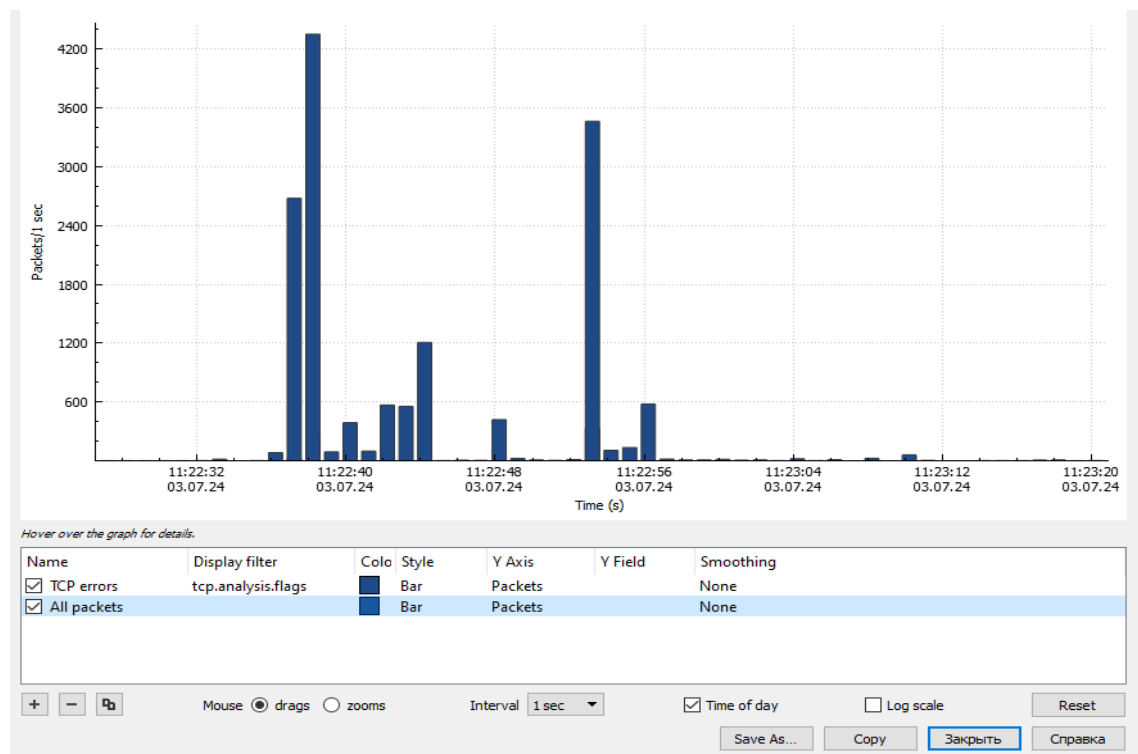
Рисунок 5.8 – Столбиковая диаграмма зависимости пропускной способности
