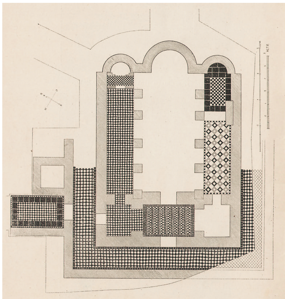
Рис. 10. Мозаичные полы Партенитской базилики. План (по: Репников Н.И. Партенитская базилика... Рис. 13)
