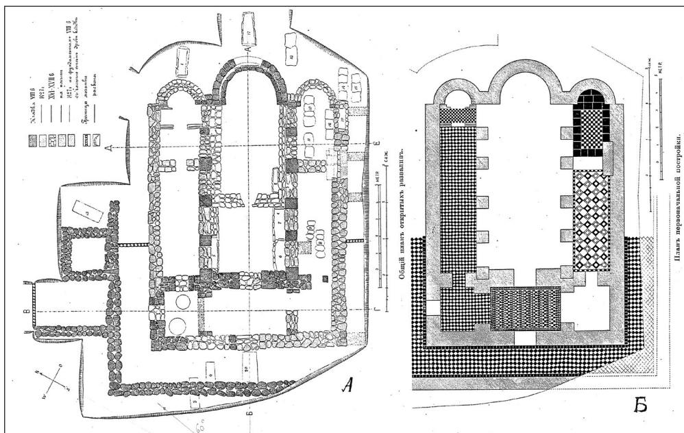
Рис. 4. План Пратенинской базилики по Н.И. Репникову (1909): А — общий план открытых развалин с прорисовкой кладок стен; Б — план первоначальной постройки с реконструкцией мозаичного пола
