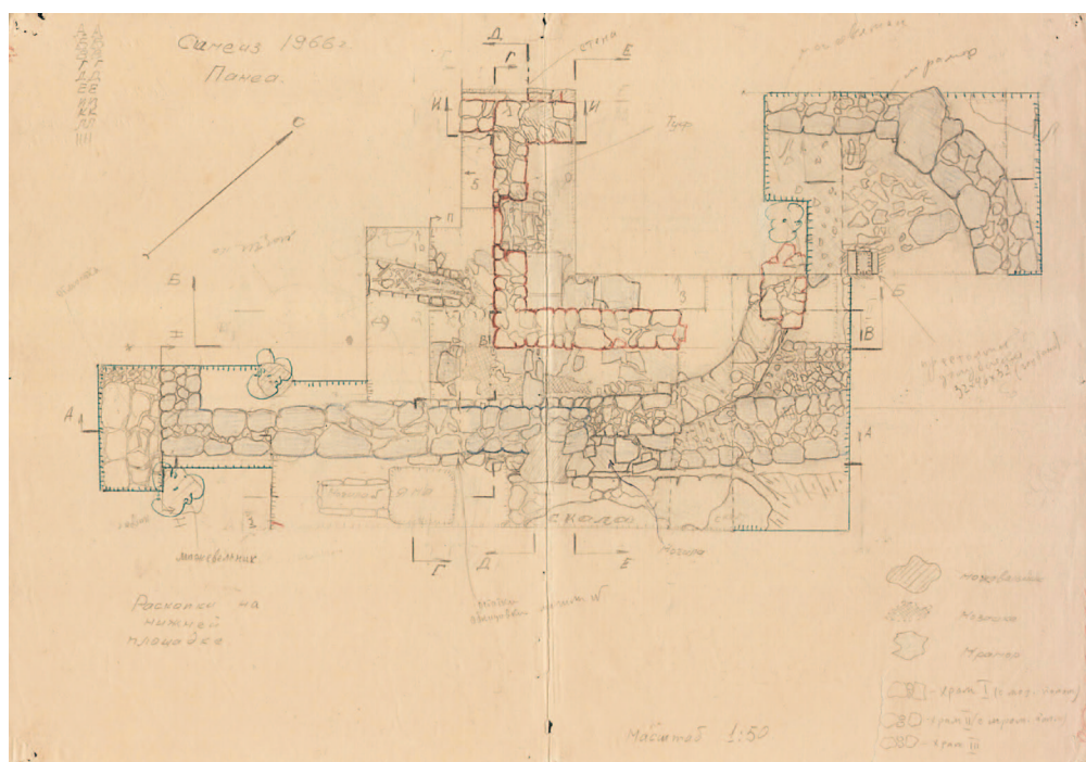
Рис. 1. Средневековые храмы Панеа. План раскопа. Обмер 1966 г. (по: Кирилло В.П. Архитектурные миграции... Рис. 11)
