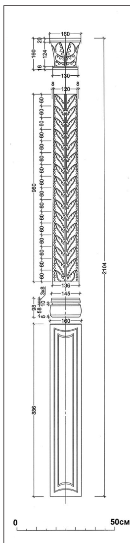
Рис. 8. Реконструкция капители, колонки, базы и столбика предaltarной преграды (выполнена архитектором А.В. Мыцом)
