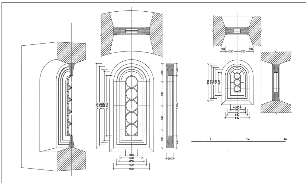
Рис. 10. Окна Партенитской базилики (реконструкция архитектора А.В. Мыца)
