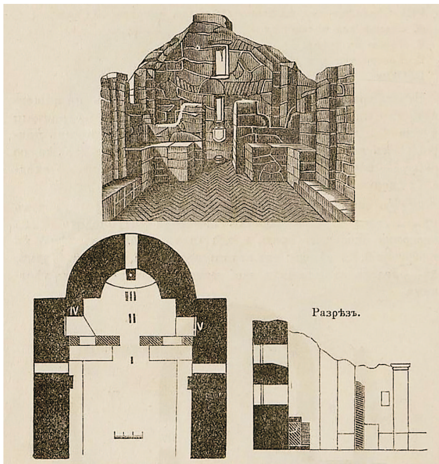
Рис. 14. Храм в Ай-Василь. Вид с запада, план и разрез (по: Струков Д. Древние памятники христианства... С. 34)
