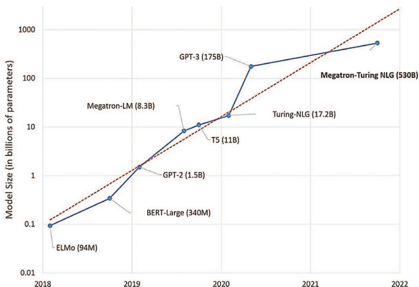
Рис. 1. Развитие БЯМ (размер моделей в миллиардах параметров) 12
