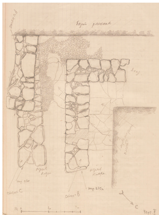
Рис. 2. Полы и кладки храмов Панеа. План. Обмер 1966 г. (по: Паршина Е.А. Разведки на скале Панеа... Л. 4 об.)
