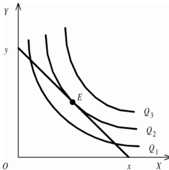
Рисунок 3 – Равновесие производителя
