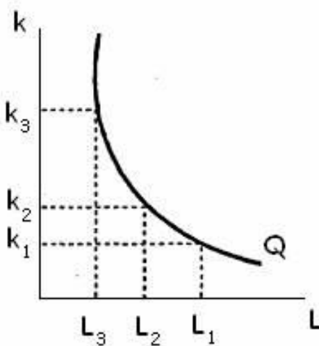
Рисунок 1 – Изокванта
