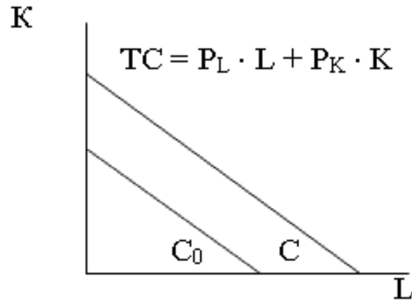
Рисунок 2 – Изокоста
