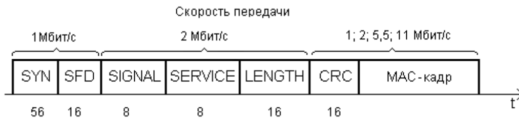
Рисунок 4 — Укороченный формат заголовка кадров сети IEEE 802.11b
