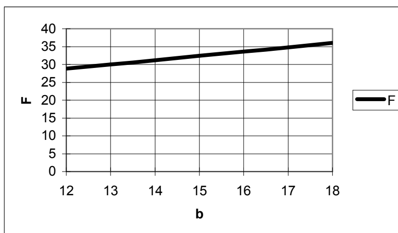
Рисунок 6.1 – Рост целевой функции при изменении запасов продукта
