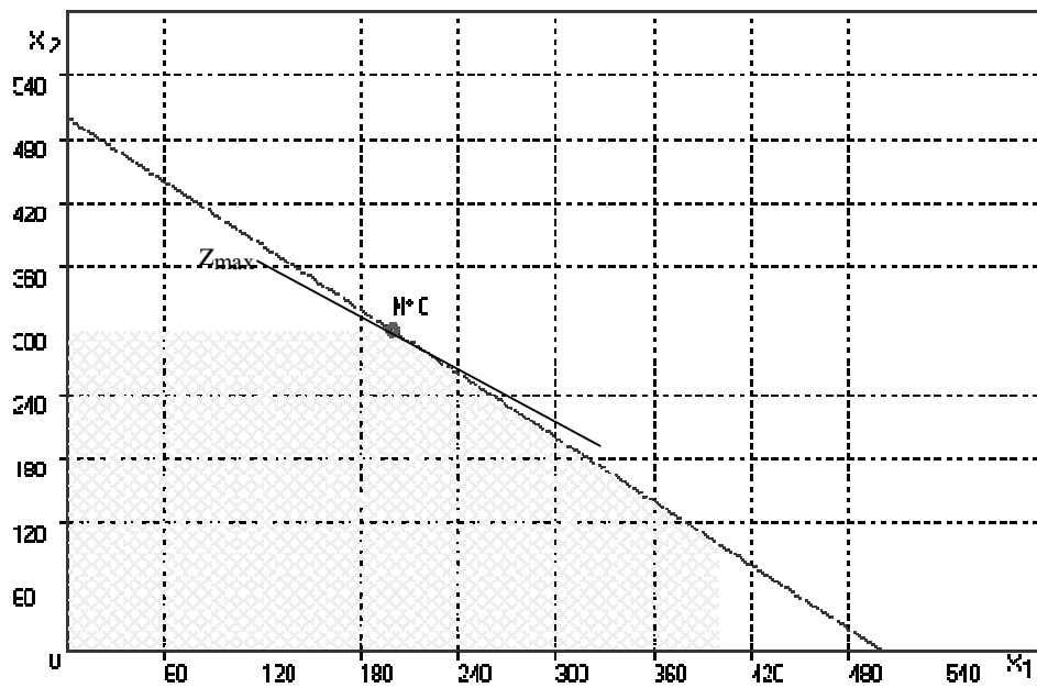
Рисунок 2.1 – Вид области допустимых решений
