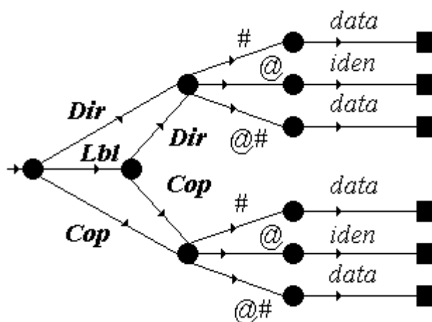
Рисунок 6.1 – Граф переходов конечного автомата при синтаксическом анализе
