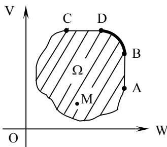
Рисунок 3.1 – Множество Парето
