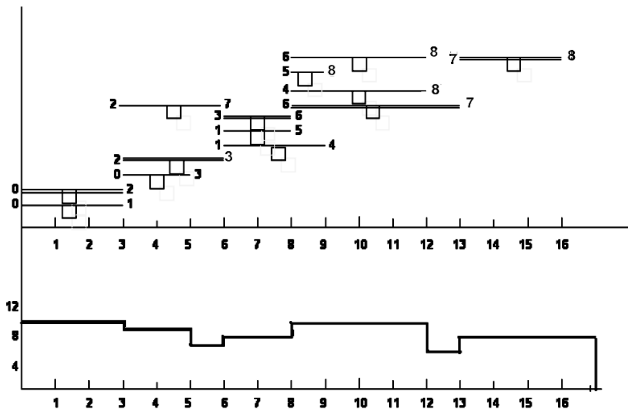
Рисунок 4.4 – Диаграмма ленточного графика и карты проекта
