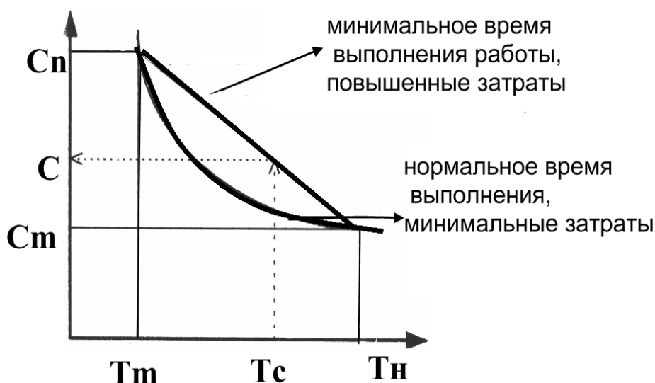
Рисунок 4.5 – График «Время - затраты»
