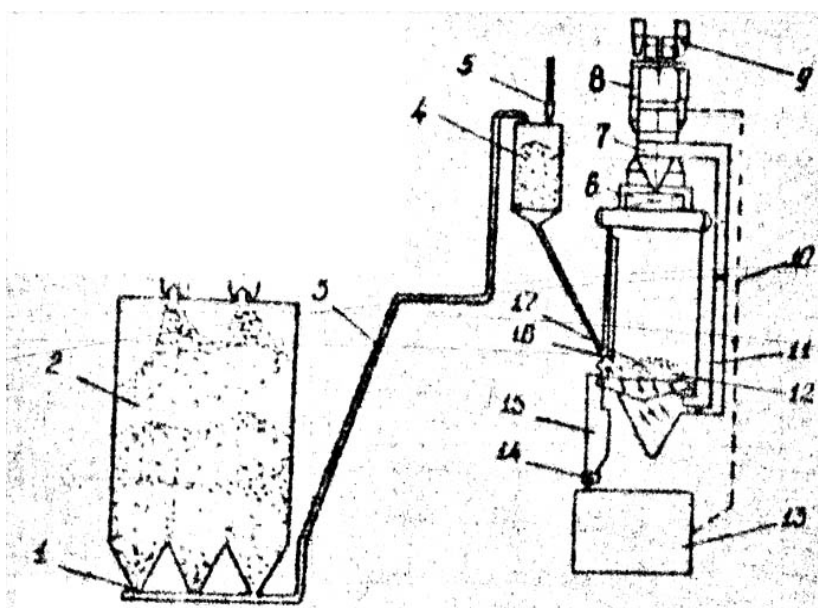
Рисунок 6.2 — Принципиальная схема системы автоматической подачи угля к котлу
