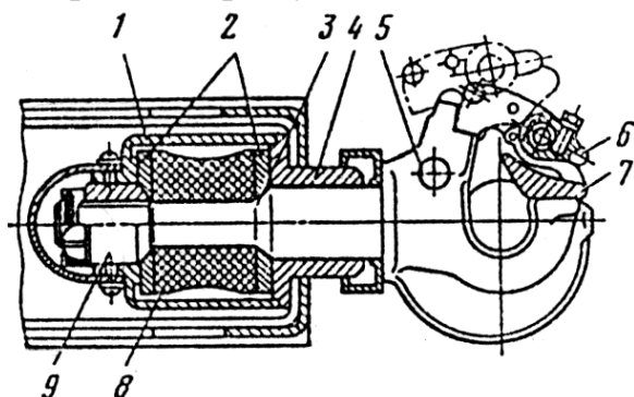
Рисунок 3.2 – Буксирный прибор
