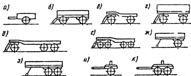
Рисунок 1.2 – Прицепы и полуприцепы:
