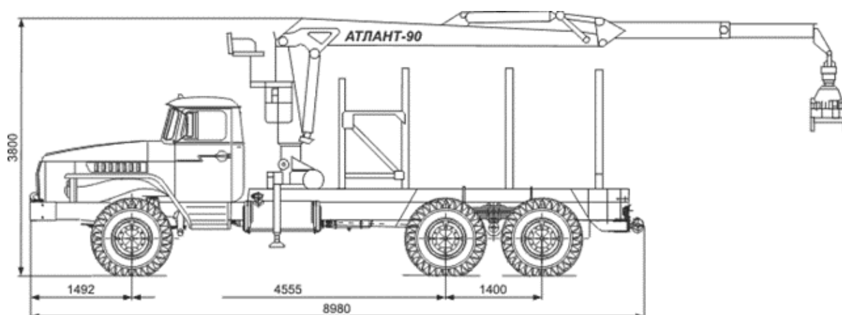
Рисунок А.5 – Сортиментовоз Урал 4320 с ГМ Атлант90
