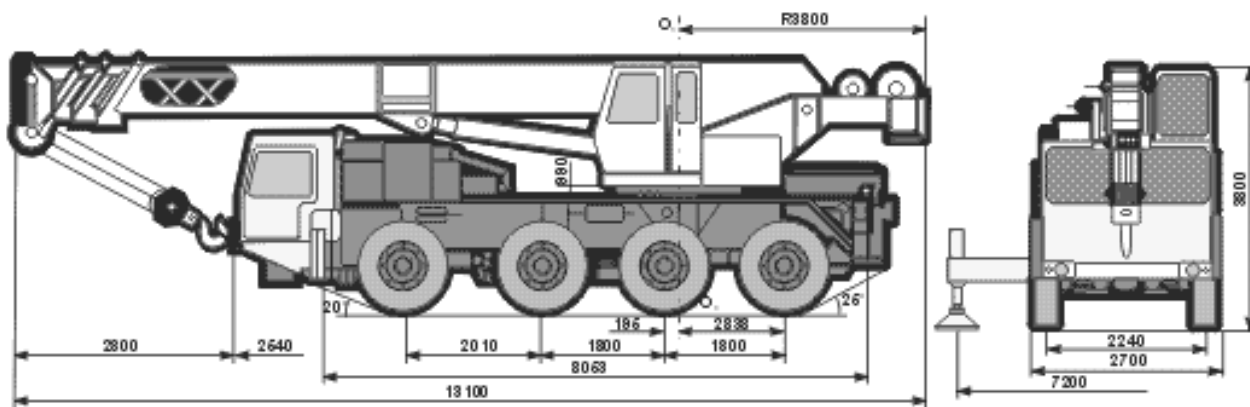
Рисунок А.3 – Кран гидравлический на специальном шасси повышенной проходимости грузоподъемностью 50 т модели КС - 6972
