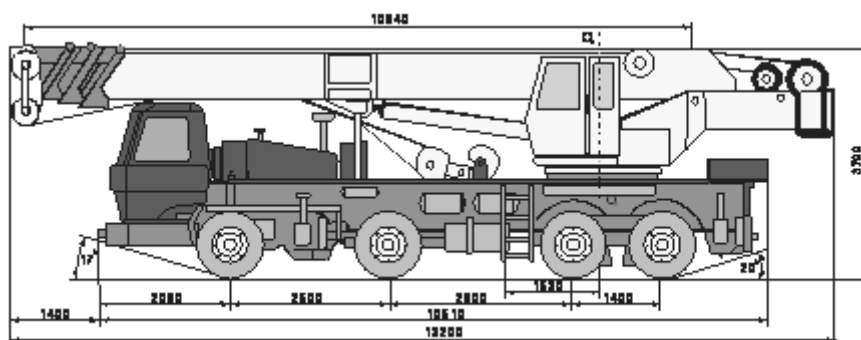
Рисунок А.6 – Кран гидравлический на специальном шасси автомобильного типа грузоподъемностью 50 т, модели КС-КШТ50.01
