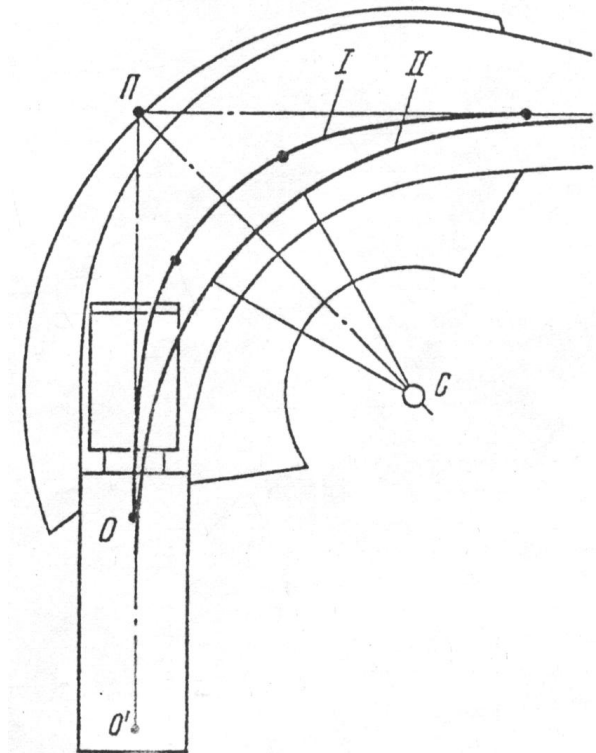
Рисунок 6.5 – Фактическая и круговая габаритные полосы движения автомобиля-тягача с полуприцепом при повороте на угол 90°: I – основная траектория середины заднего моста автомобиля-тягача; II – траектория задней оси полуприцепа; продольная ось автомобиля-тягача; C – центр поворота
