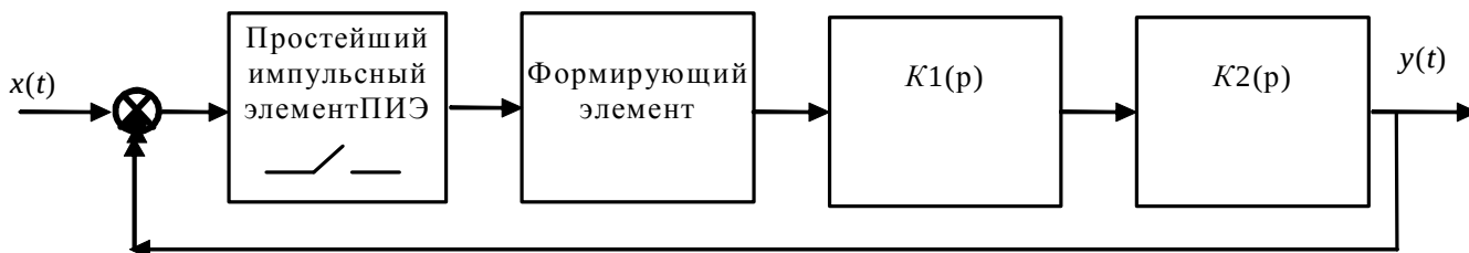
Рис. 5.1 — Структурная схема системы
