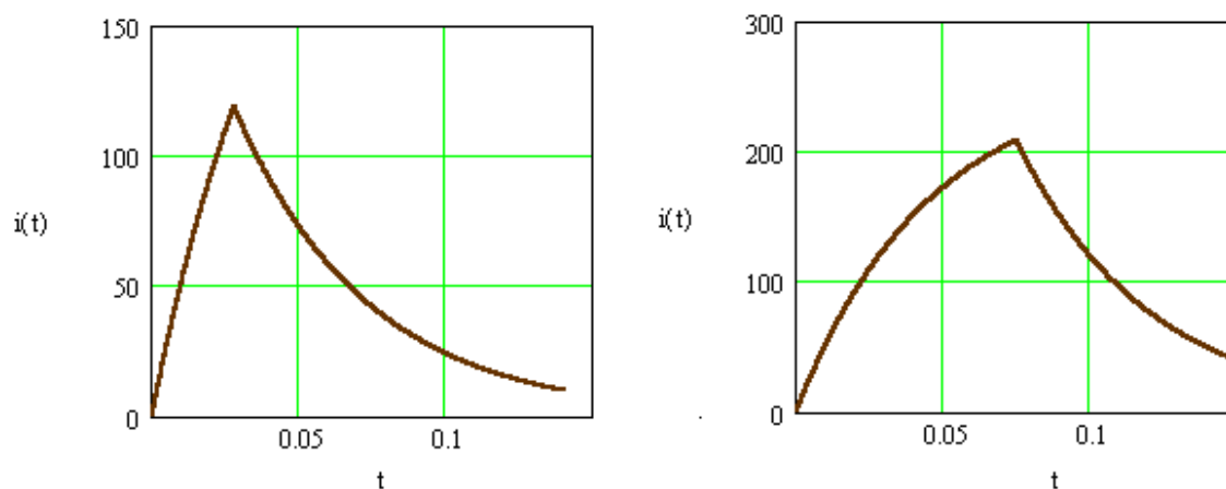
Рисунок 4 – Осциллограммы рабочего тока в соленоиде при его непосредственном подключении к источнику постоянного напряжения и различной длительности импульса тока
