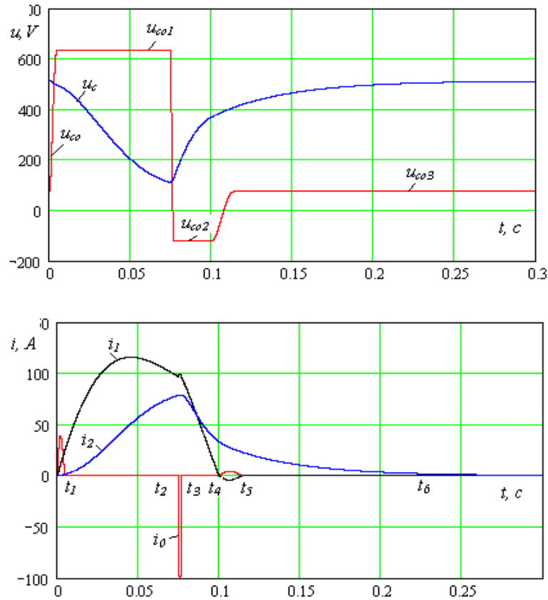
Рисунок 2 – Осциллограмма напряжений и токов конденсаторной схемы электропитания
