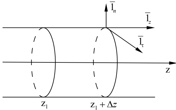
Рисунок 5.8 — К расчету затухания электромагнитной волны в волноводe
