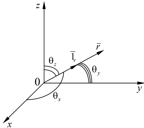
Рисунок 4.2 — К выводу уравнения волны, движущейся в произвольном направлении
