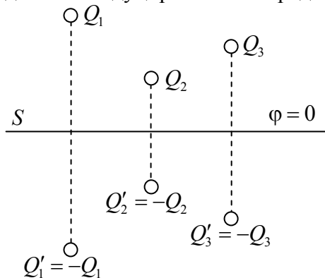
Рисунок 2.2 — К расчету поля зарядов над проводящей поверхностью
