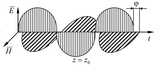
Рисунок 3.2 — Векторы \vec{E} и \vec{H} в среде с потерями
