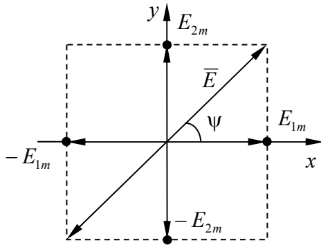
Рисунок 3.5 — К определению линейно поляризованной волны
