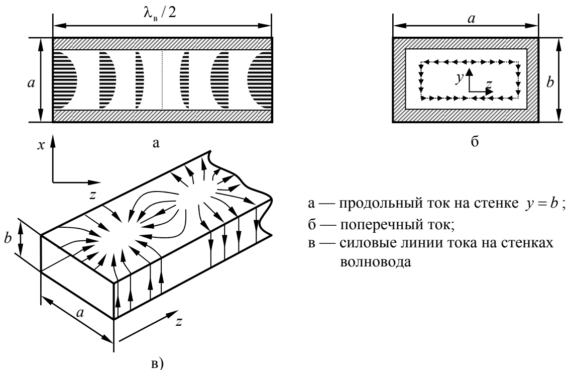
Рисунок 5.4 — Токораспределение на стенках волновода с волной H_{10}
