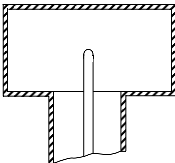
Рисунок 5.7 — Возбуждение волны H_{10} в прямоугольном волноводe с помощью штыря
