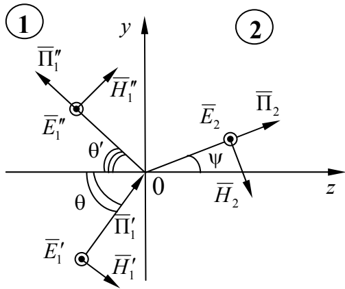
Рисунок 4.3 — Векторы поля на границе раздела сред при наклонном падении (перпендикулярная поляризация)
