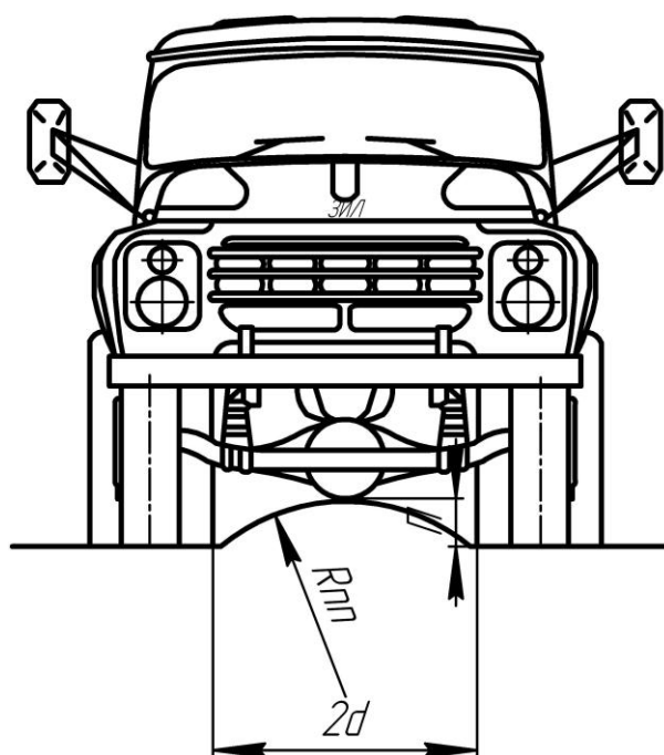
Рисунок 9.3 – Поперечный радиус проходимости
