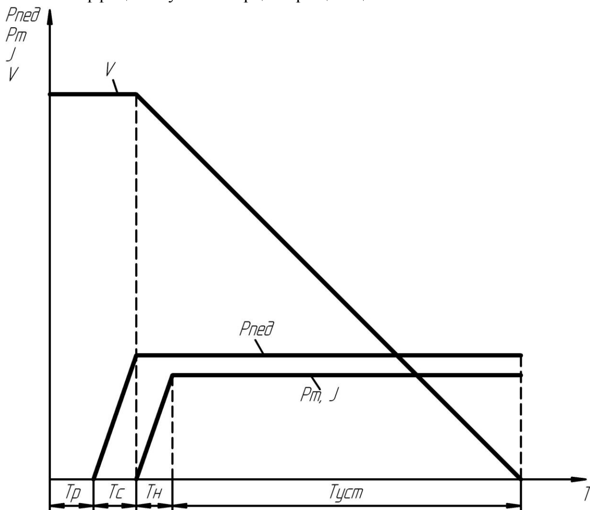
Рисунок 8.1 – Тормозная характеристика автомобиля
