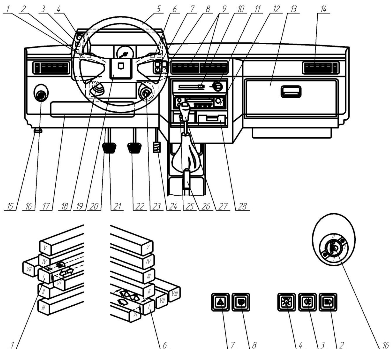
Рисунок 2.1 – Органы управления автомобиля ЗАЗ-11026
