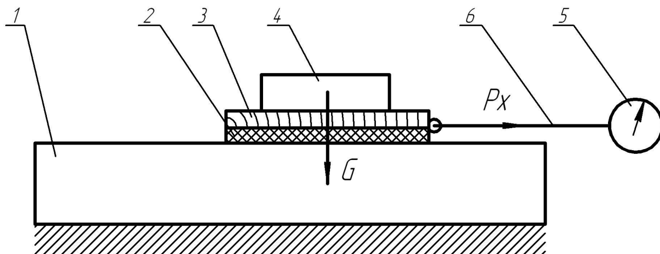
Рисунок 3.2 – Схема лабораторной установки
