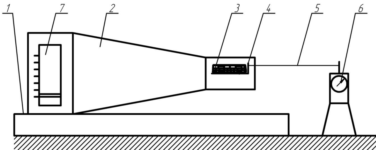
Рисунок 6.2 – Аэродинамическая труба
