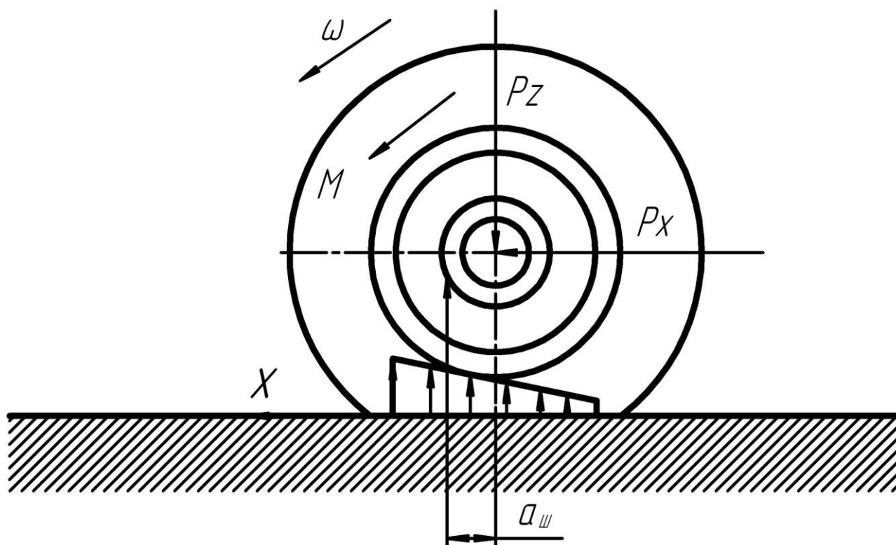
Рисунок 4.1 – Гистерезисные потери в шине
