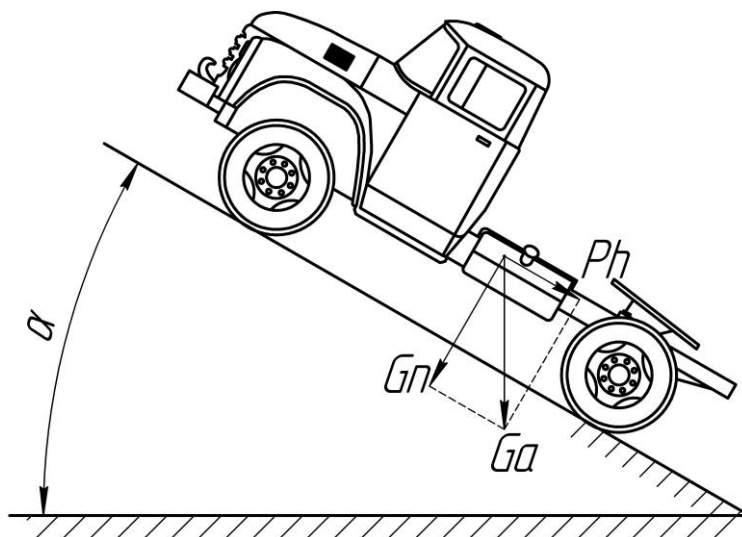
Рисунок 9.4 – Силы, действующие на автомобиль во время подъема
