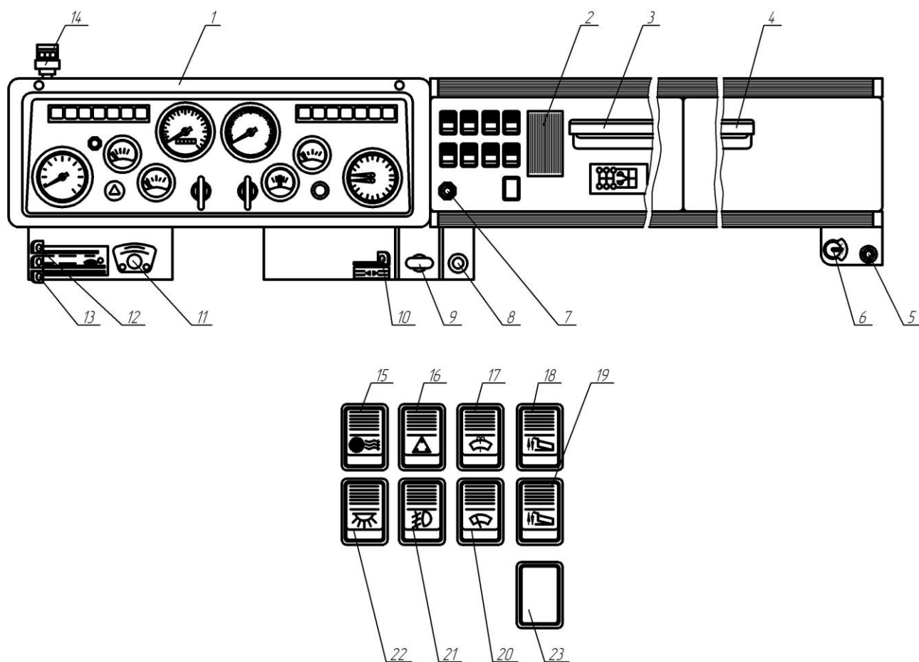
Рисунок 2.7 – Панель контрольно-измерительных приборов автомобиля семейства КамАЗ
