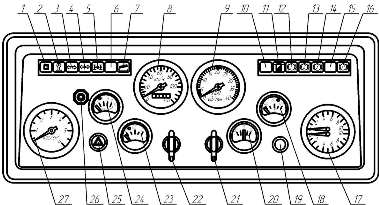
Рисунок 2.6 – Комбинация приборов автомобиля семейства КамАЗ
