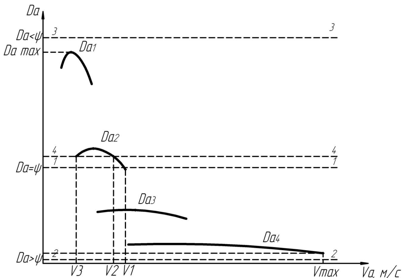
Рисунок 7.1 – Динамическая характеристика автомобиля
