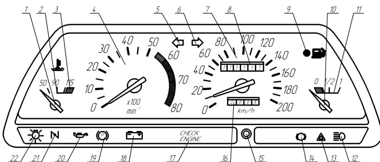
Рисунок 2.4 – Комбинация приборов легкового автомобиля ВАЗ-2110
