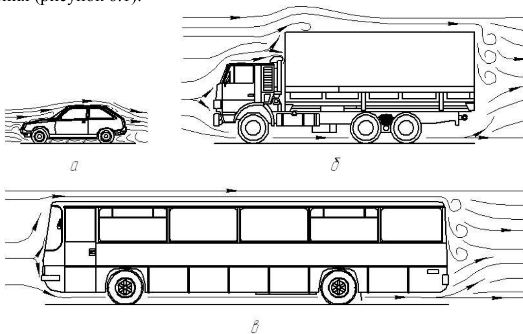
Рисунок 6.1 – Направление воздушных потоков:
