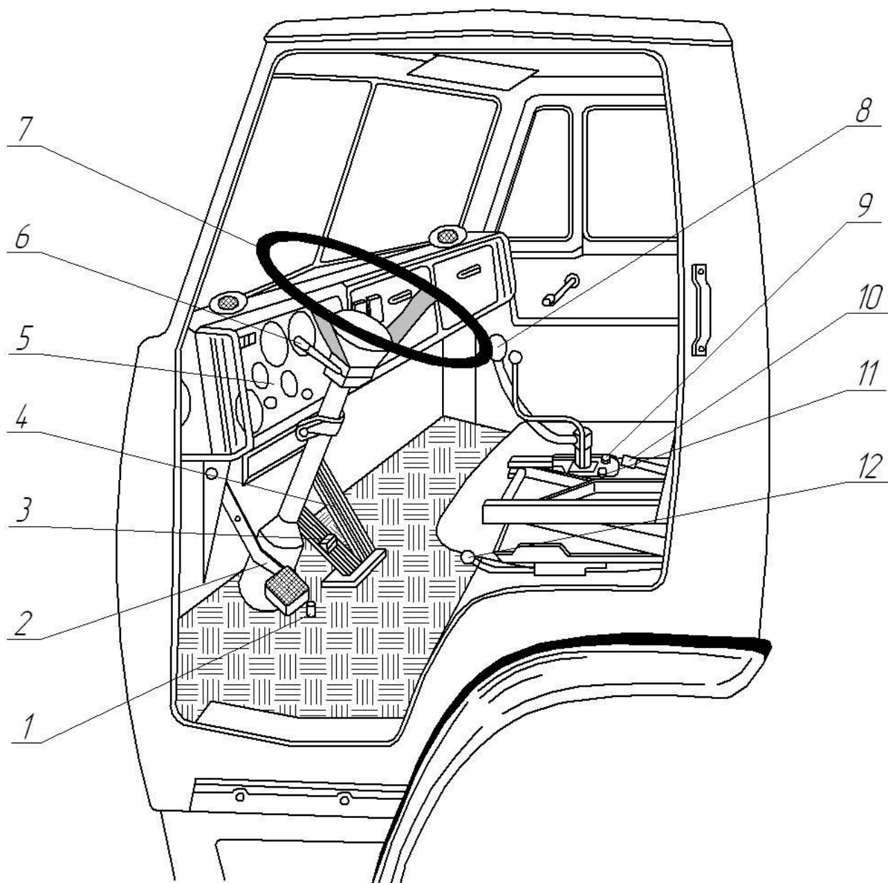
Рисунок 2.5 – Органы управления автомобиля семейства КамАЗ
