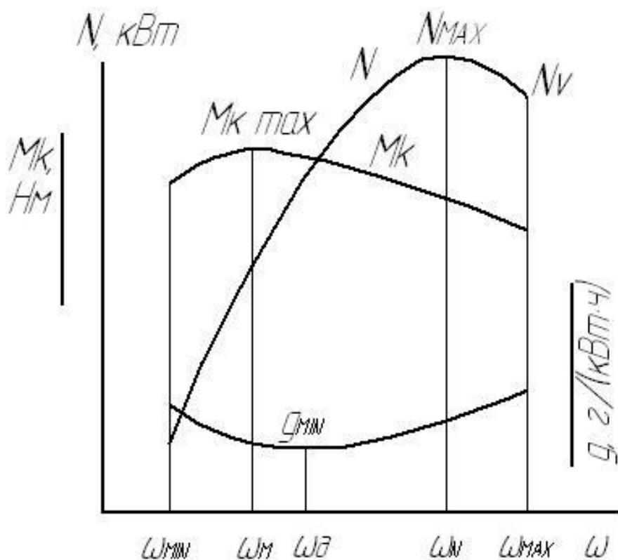
Рисунок 7.2 – Внешняя скоростная характеристика карбюраторного двигателя легкового автомобиля без ограничителя частоты вращения
