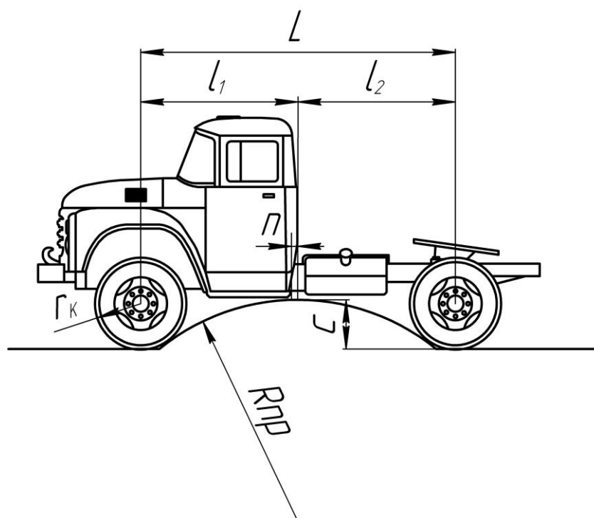
Рисунок 9.2 – Продольный радиус проходимости
