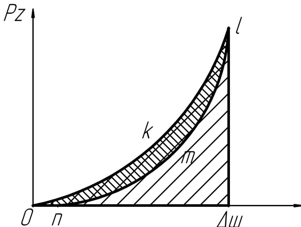
Рисунок 4.1 – Гистерезисные потери в шине
