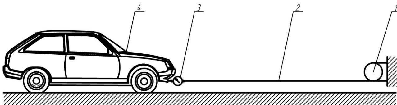
Рисунок 4.4 – Схема проведения экспериментов
