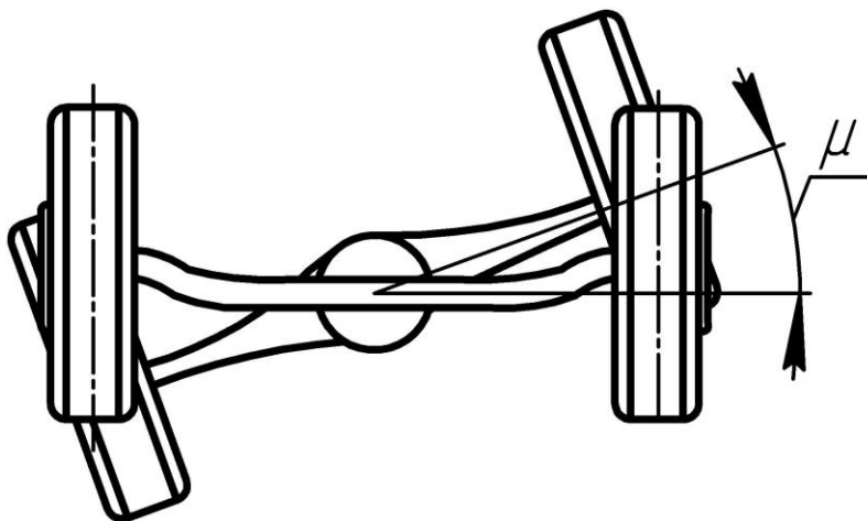
Рисунок 9.4 – Угол перекоса осей автомобиля
