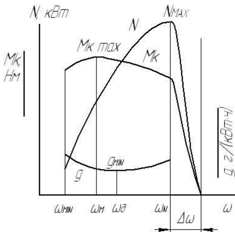
Рисунок 7.4 – Внешняя скоростная характеристика дизельного двигателя
