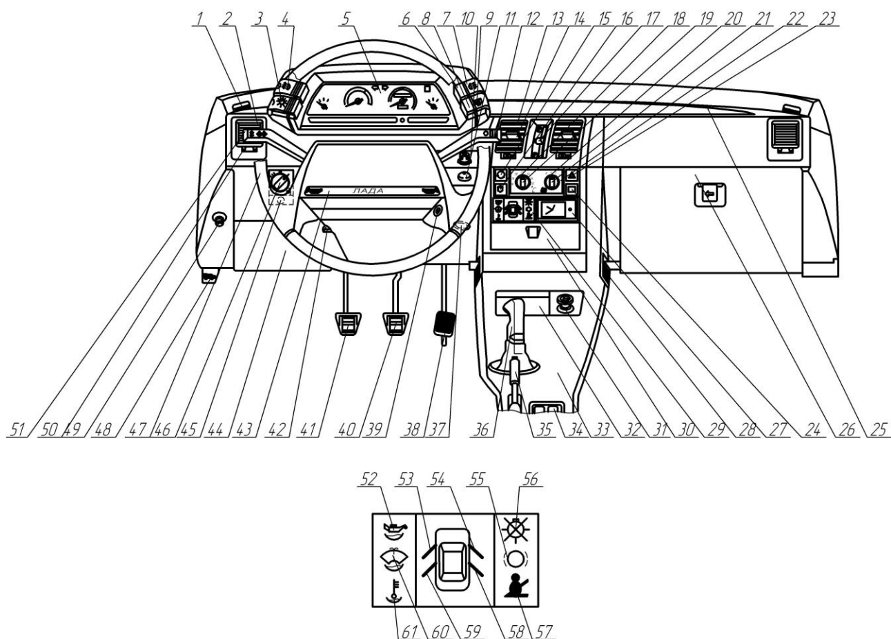
Рисунок 2.3 – Органы управления легкового автомобиля ВАЗ-2110
