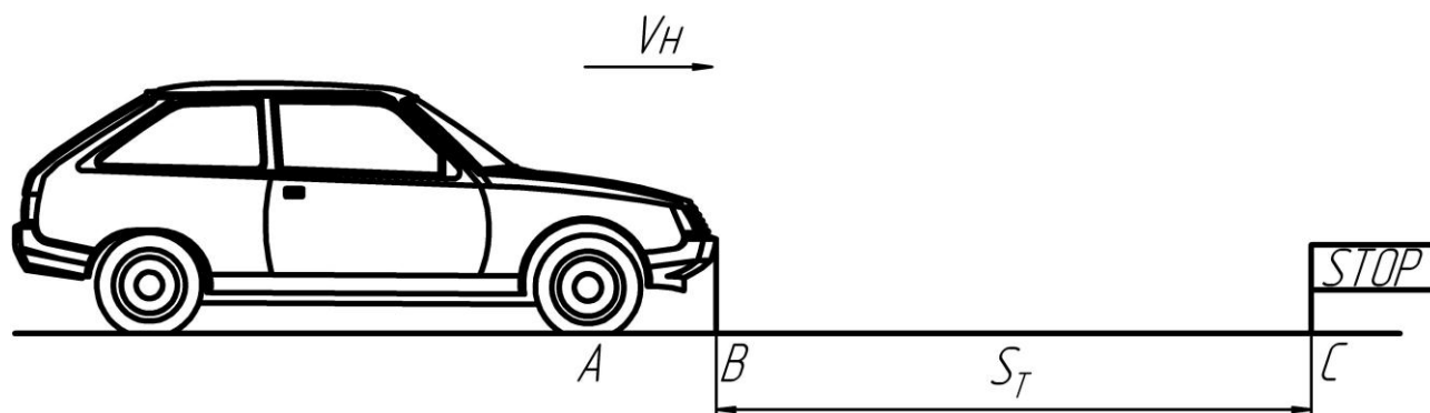
Рисунок 8.2 – Схема проведения эксперимента
