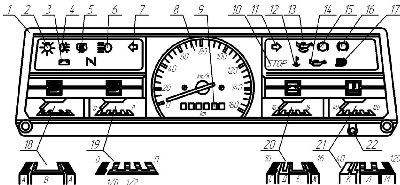
Рисунок 2.2 – Комбинация приборов автомобиля ЗАЗ-11026
