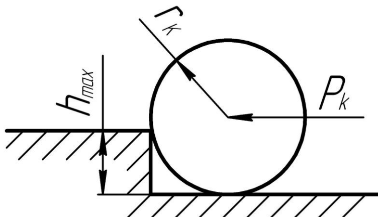
Рисунок 9.1 – Преодоление колесом пороговых препятствий
