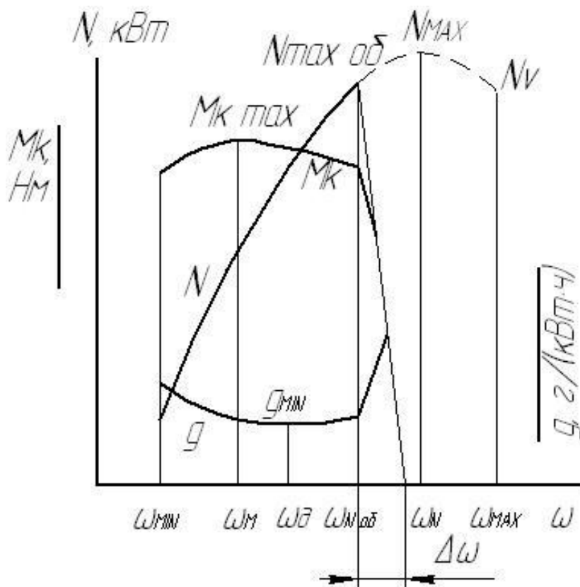
Рисунок 7.3 – Внешняя скоростная характеристика карбюраторного двигателя легкового автомобиля с ограничителем частоты вращения
