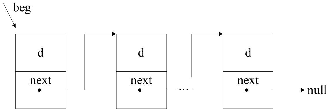
Рисунок 3.1 — Линейный список
