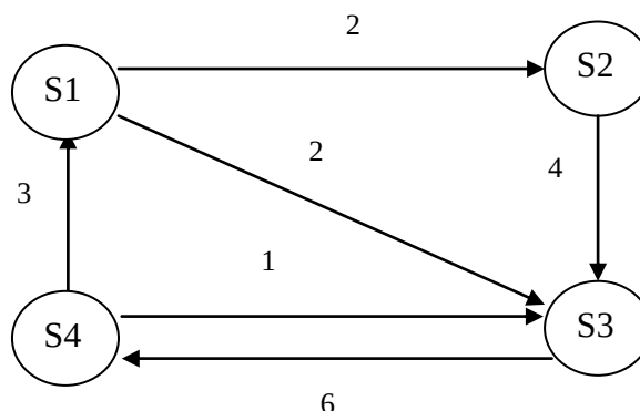
Рисунок 1.3 – Граф переходов непрерывной марковской цепи
