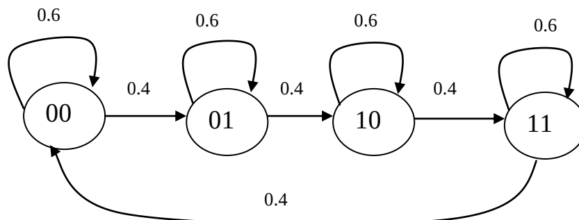
Рисунок 1.2 – Граф переходов дискретной марковской цепи
