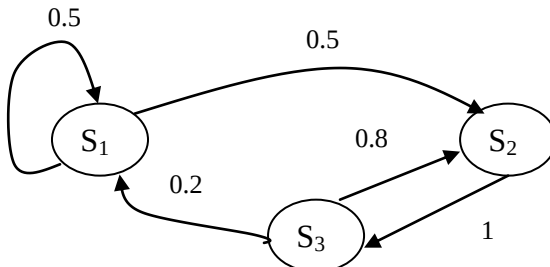
Рисунок 1.1 – Граф переходов дискретной марковской цепи
