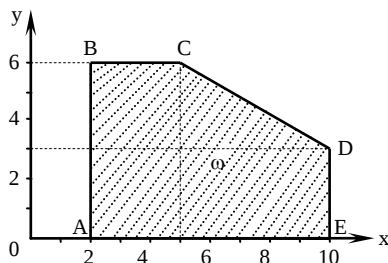
Рисунок 3.4 – Множество \omega
