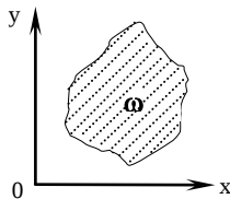
Рисунок 3.2 – Множество \omega
