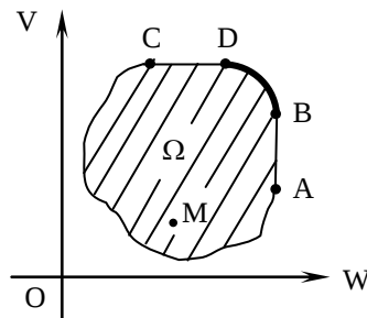
Рисунок 3.1 – Множество Парето
