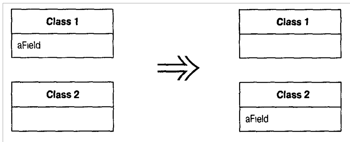
Рисунок 2.2 – Перемещение поля
