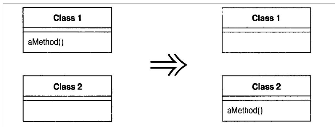
Рисунок 2.1 – Перемещение метода
