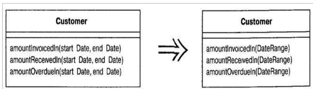
Рисунок 2.9 – Введение граничного объекта
