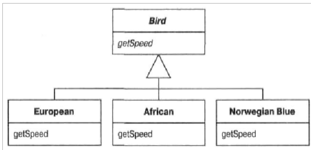
Рисунок 2.1 – Замена условного оператора полиморфизмом
