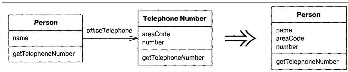
Рисунок 2.4 – Встраивание класса
