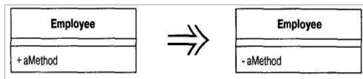
Рисунок 2.11 – Соккрытие метода
