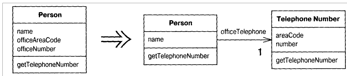
Рисунок 2.3 – Выделение класса
