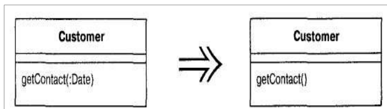
Рисунок 2.3 – Удаление параметра
