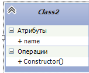
Рис. 2 – Абстрактный класс.
