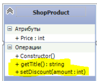
Рис. 5 – Операции класса в нотации UML.
