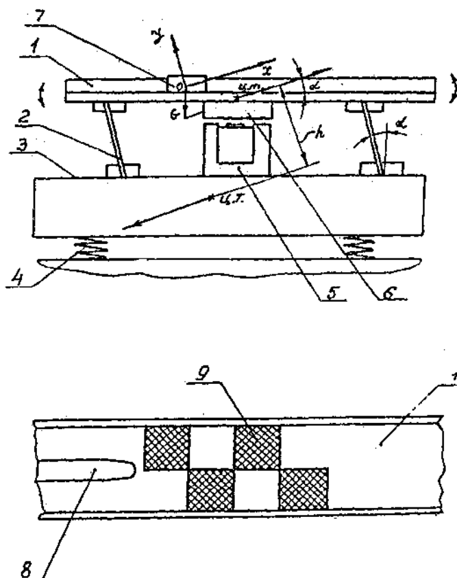
Рисунок 1 - Вибролоток
