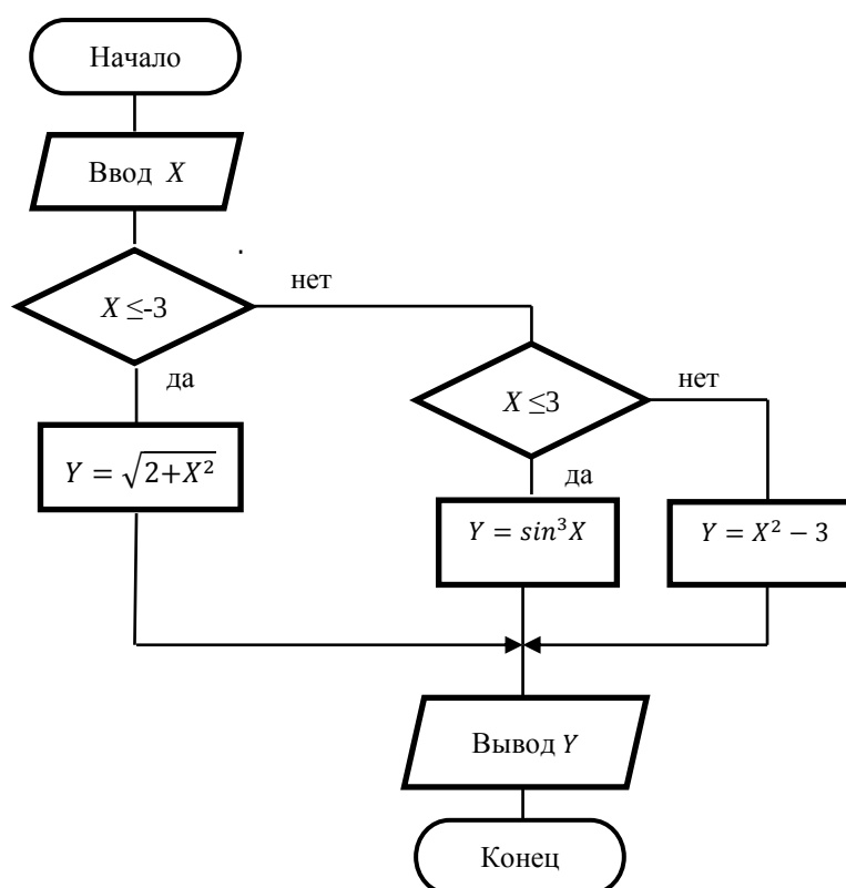
Рис. 4.1. - Схема алгоритма
