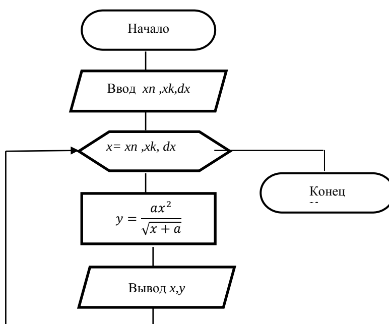
Рис. 5.1. - Схема алгоритма
