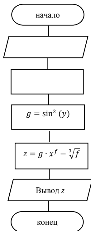
Рис. 3.1 - Схема алгоритма
