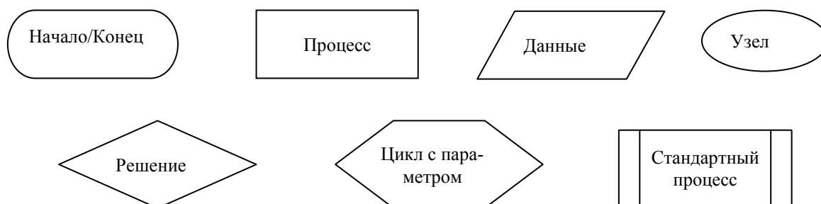
Рис. 1.1 - Элементы блок-схемы
