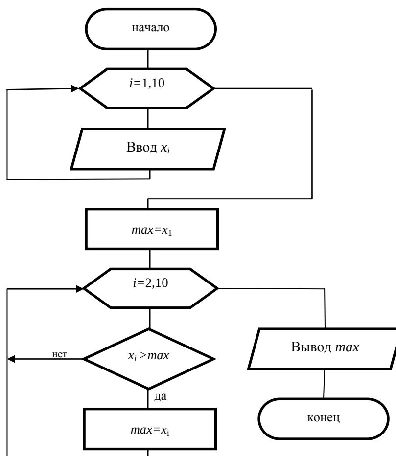
Рис. 6.2 – Схема алгоритма
