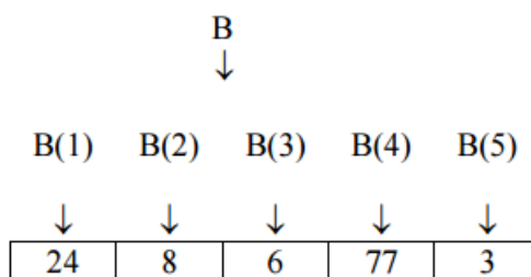
Рис. 6.1 – Одномерный массив из пяти элементов
