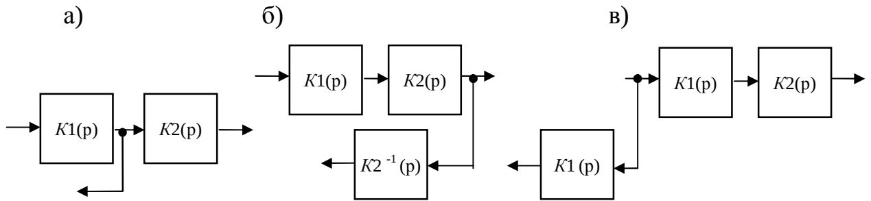
Рис. 1.4 — Преобразования звеньев СРА: исходная схема (а), при переносе ветви по направлению прохождения сигнала (б), при переносе ветви против прохождения сигнала (в)
