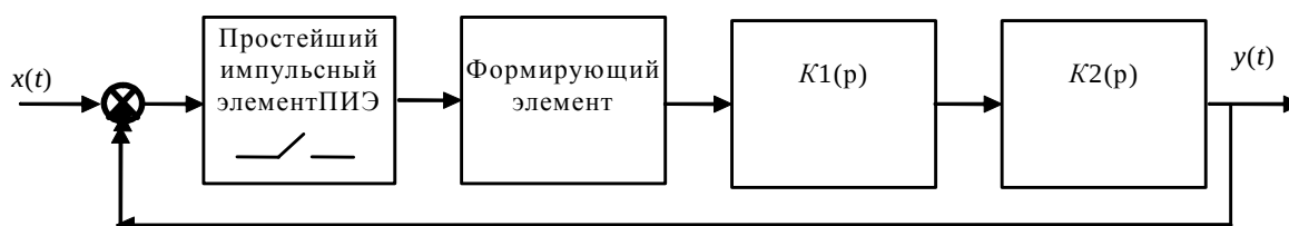
Рис. 5.1 — Структурная схема системы 4
