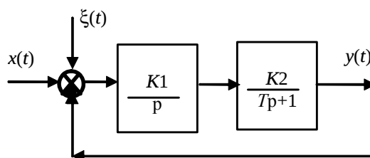
Рис. 4.1 — Структурная схема системы 3
