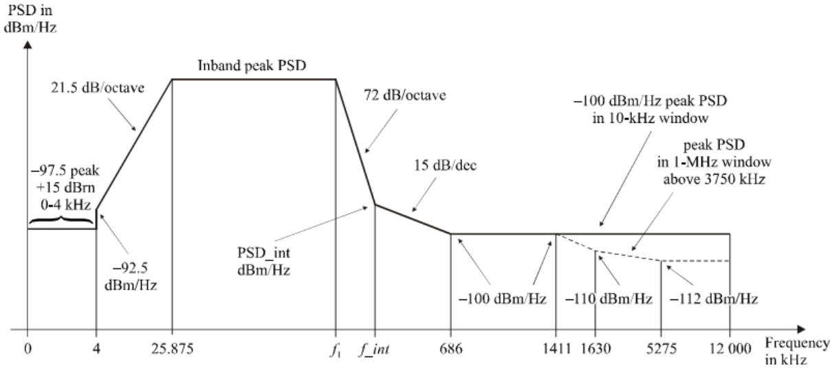
Рис. 1.6 — Спектральная маска для передатчика модема ADSL2+
