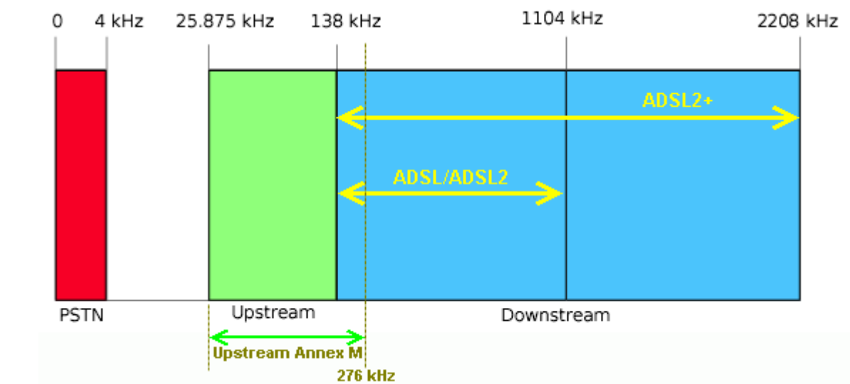
Рис. 1.5 — Схема использования диапазона частот ADSL , ADSL2 и ADSL2+
