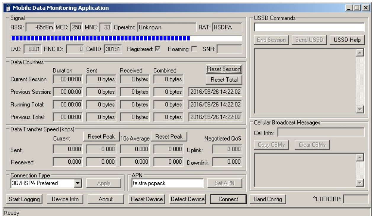
Рис. 3.10 — Основное окно программы MDMA
