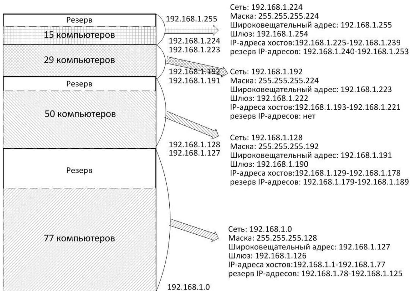
Рисунок 1.6 – Пример планирования IP-адресов для четырех подсетей
