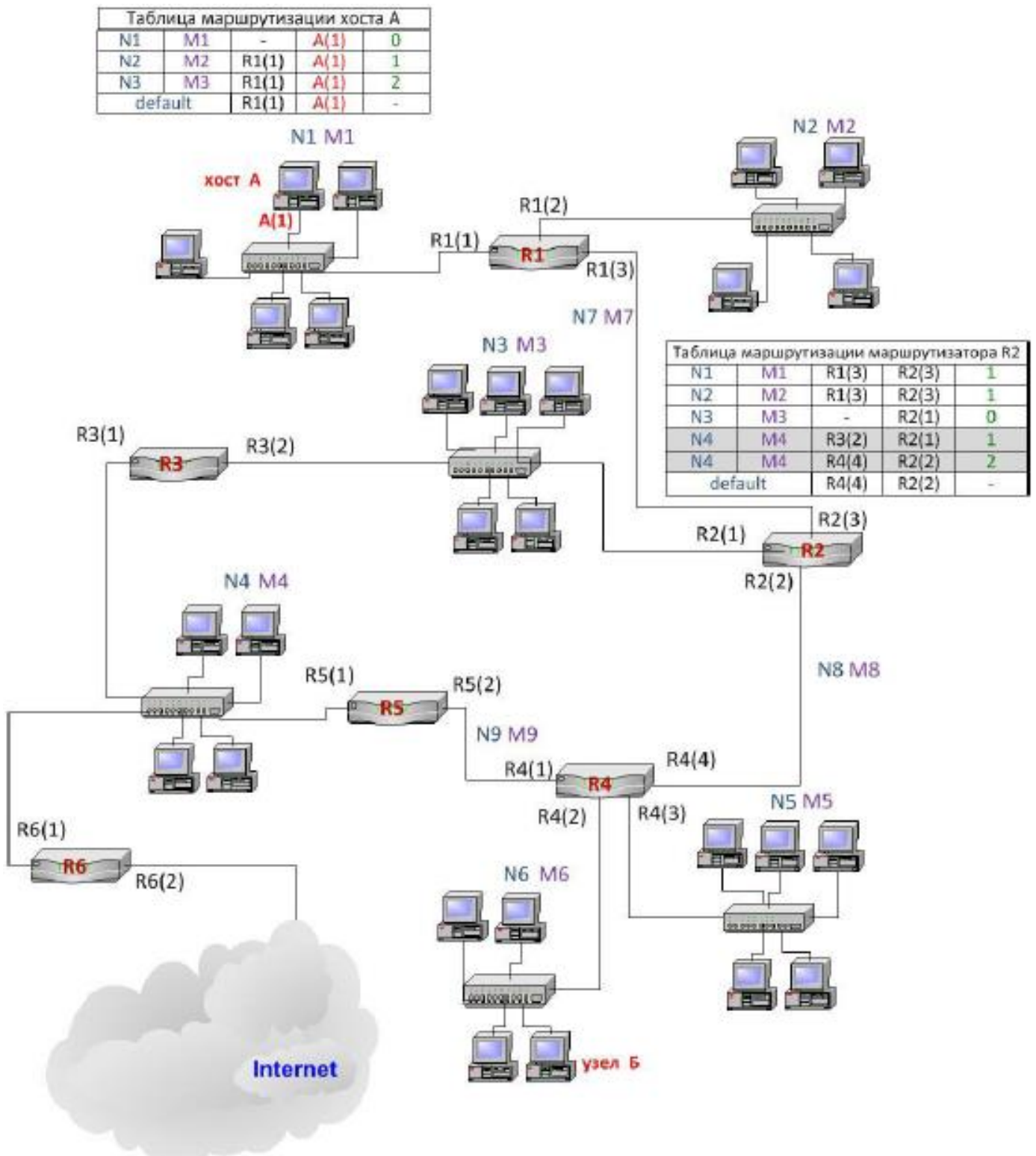
Рисунок 1.9 – Маршрутизация в составной сети
