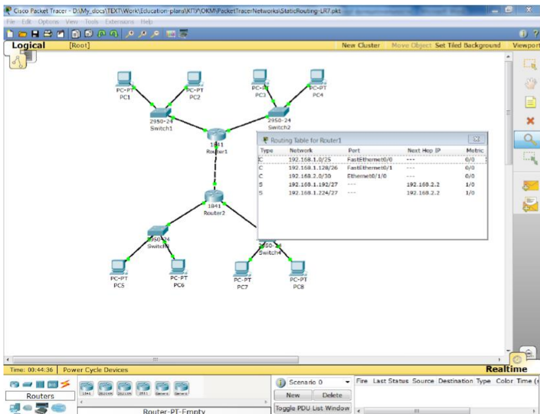
Рисунок 1.14 – Просмотр таблицы маршрутизации маршрутизатора
