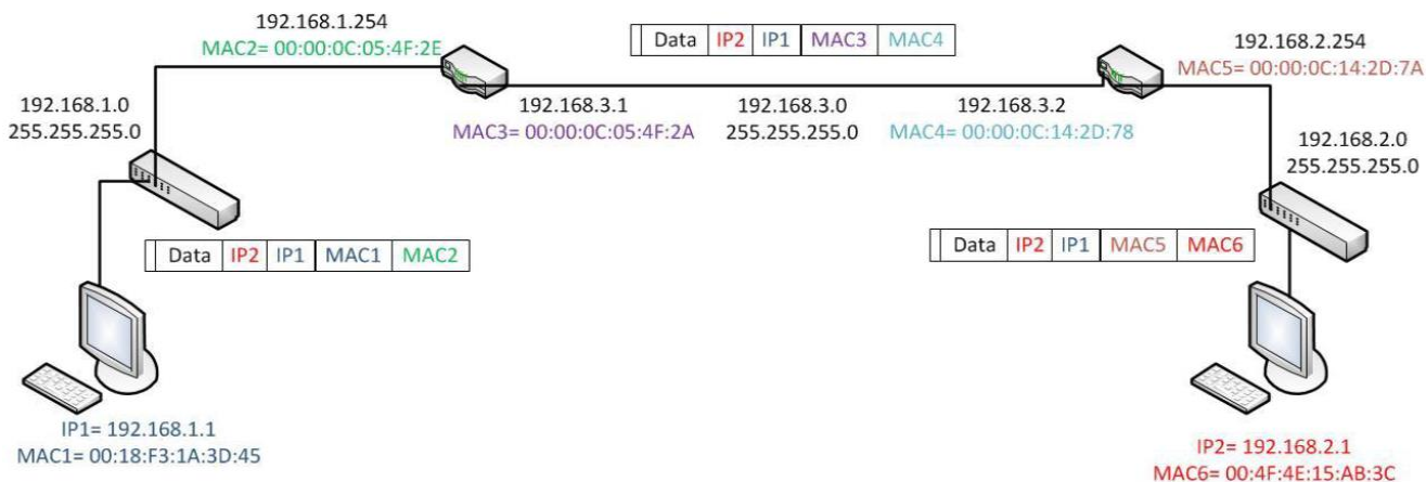
Рисунок 1.11 – Изменение адресов канального уровня при передаче дейтаграммы в составной сети.
