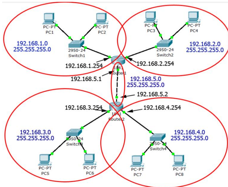
Рисунок 1.1 – Пример составной IP-сети
